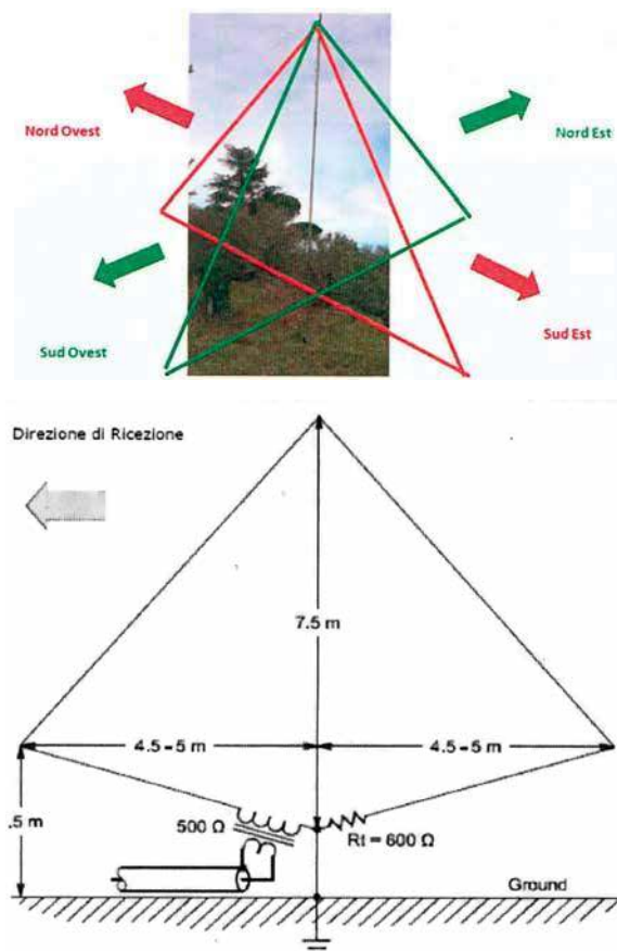
Rys. 3. Szkic pętli anteny Loop K9AY
