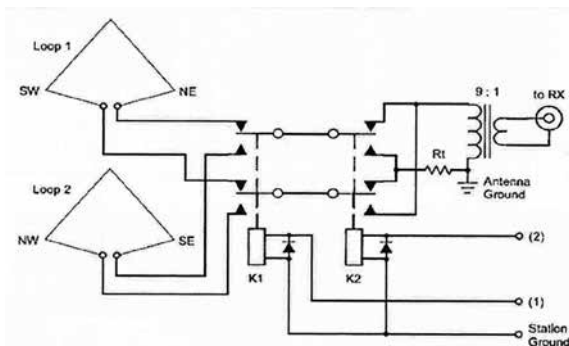
Rys. 4. Schemat przełącznika przekąźnikowego
