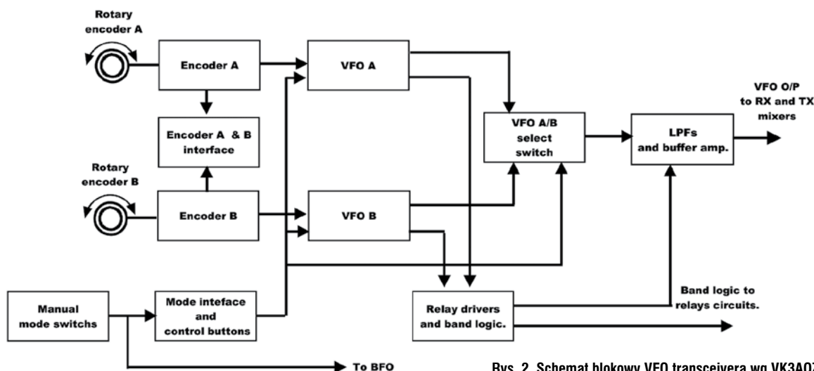
Rys. 2. Schemat blokowy VFO transceivera wg VK3AQZ
