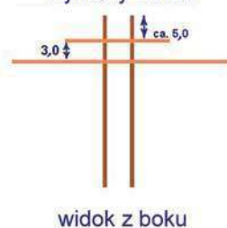
Rys. 19. Wymiary anteny planarnej na pasmo 13 cm. Elementy są wykonane z blachy mosiężnej lub miedzianej o grubości 1 mm, a falowód środkowy z rurki miedzianej o średnicy zewnętrznej 22 mm i wewnętrznej 20 mm. Do punktu zasilania podłączony jest kontakt środkowy gniazdka koncentrycznego. Należy stosować gniazdka dobrej jakości z kołnierzem montażowym i izolatorem teflonowym
