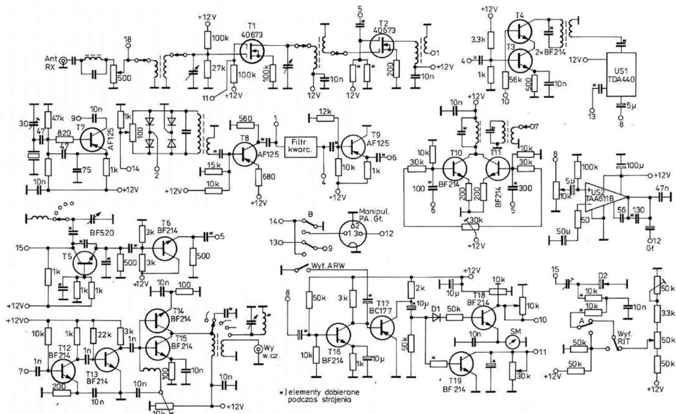
Rys. 2. Schemat zasadniczej części transceivera Jowisz SP102
