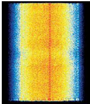
Rys. 2. Widmo sygnału P25 z kluczkowaniem CQPSK
