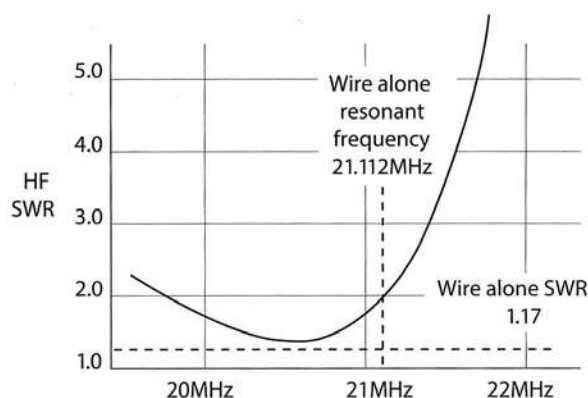
Rys. 8. Wybrana charakterystyka SWR anteny
