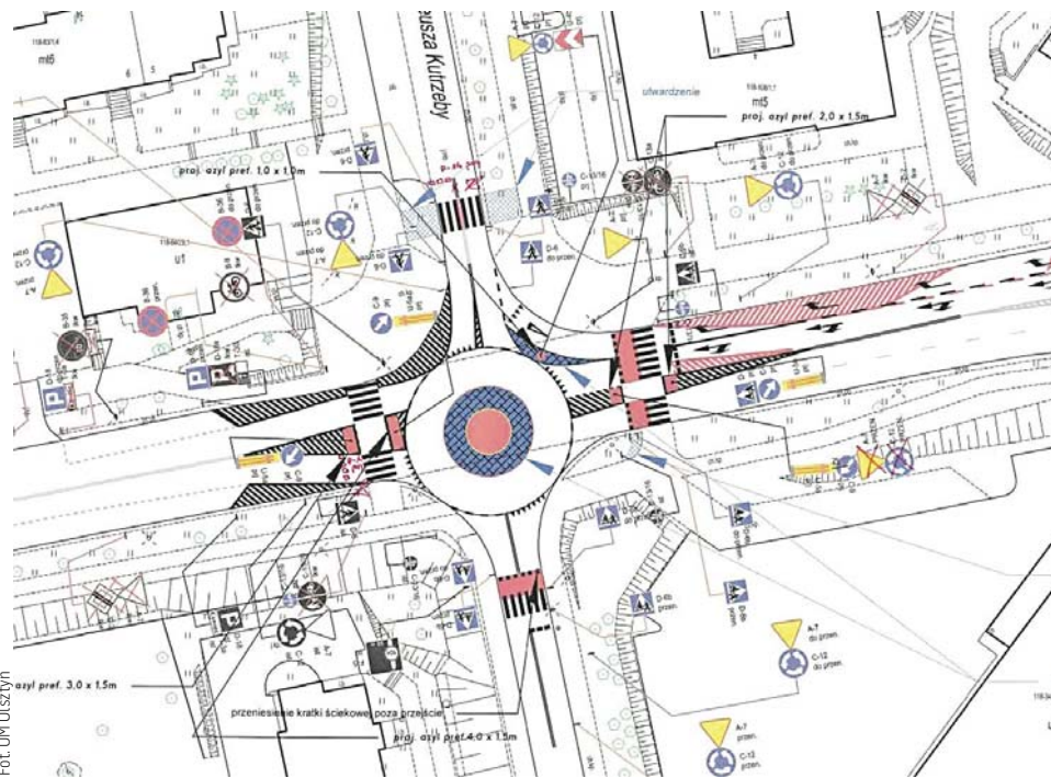
Schemat nowej organizacji w okolicach ronda Wilczyńskiego/Kutrzeby/Barcza
