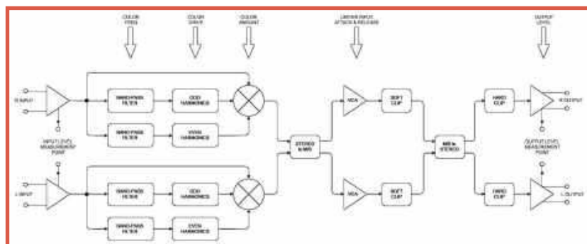
Struktura toru sygnałowego uwzględnia konwersję stereo do Mid-Side przed układem clippera i ponowną konwersję do stereo przed finalnymi ogranicznikami.
