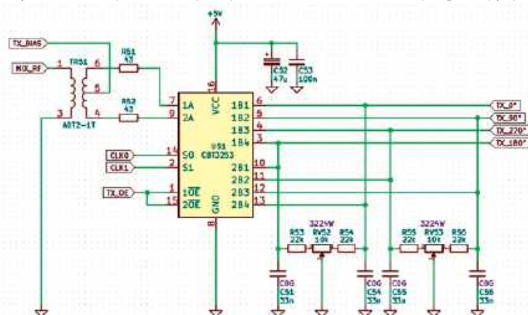
Rys 1. Schemat modulatora Tayloe z równoważeniem kluczy potencjometrami montażowymi
