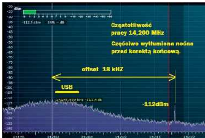
Rys 11. Pomiar poziomu wytłumienia nośnej przed ostateczną korektą potencjometrów. Test w paśmie 20 MHz
