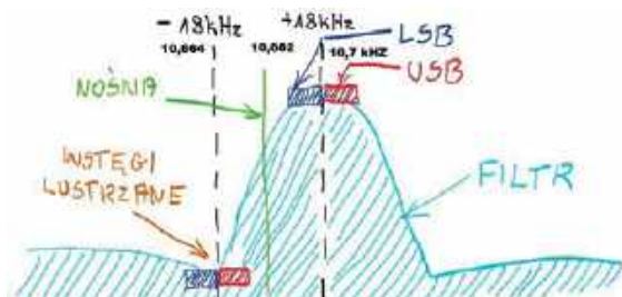
Rys 6. Sygnały LSB i USB wytworzone w modulatorze Tayloe w filtrze 10,7MHz
