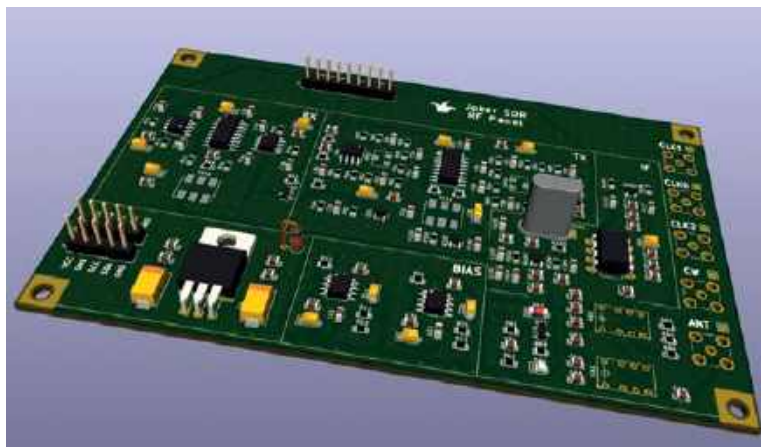
Projekt płytki mieszczącej modulator Tayloe, tor pośredniej częstotliwości z mieszaczem nadajnika
