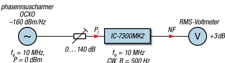
Rys. 3. Pomiar zakresu dynamiki ograniczonego przemianą wsteczną (RMDR) i szumów generatora taktującego (SBN)
