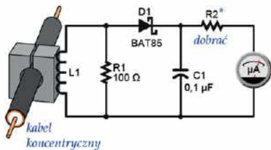
Rys. 1. Schemat ideowy amperomierza w.cz. Cewka L1 nawinięta na zatrzaśkiwanym rdzeniu ferrytowym składa się z 10 zwojów cienkiego drutu. Po zatrzaśnięciu rdzenia powstaje transformator prądowy o dużej przekładni. Natężenie prądu powierzchniowego jest odczytywane na mikroamperomierzu po jego wyprostowaniu za pomocą diody D1. Opornikiem R2 nastawiana jest czułość miernika
