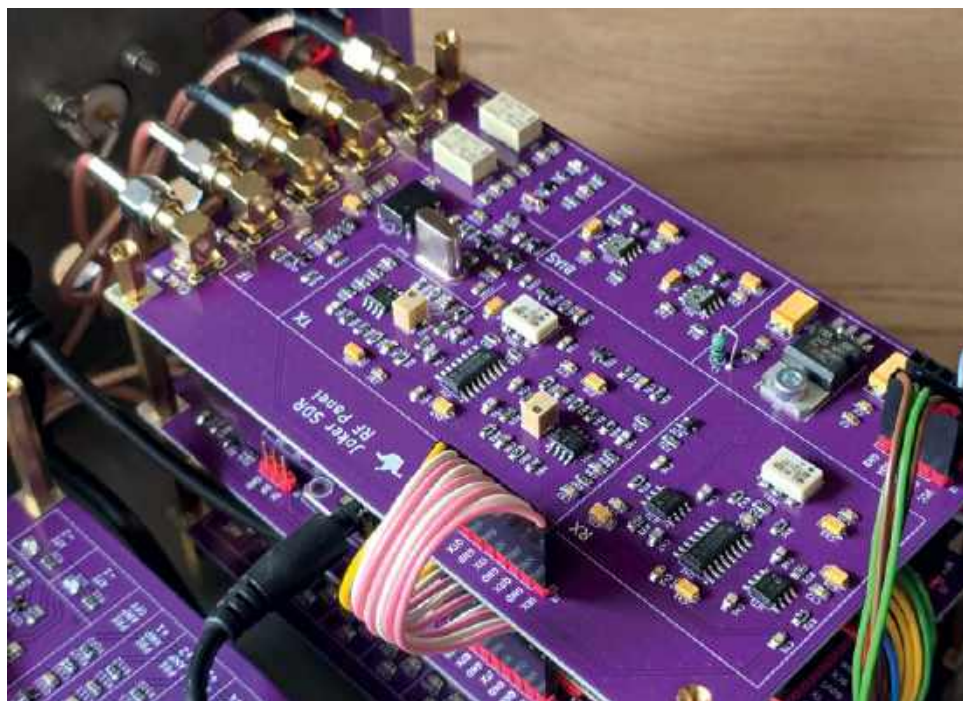
Widok zmontowanego toru pośredniej częstotliwości układu hybrydowego
