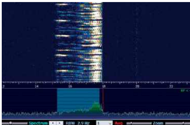
Rys 4. Uformowana dolna wstęga boczna poniżej 18kHz
