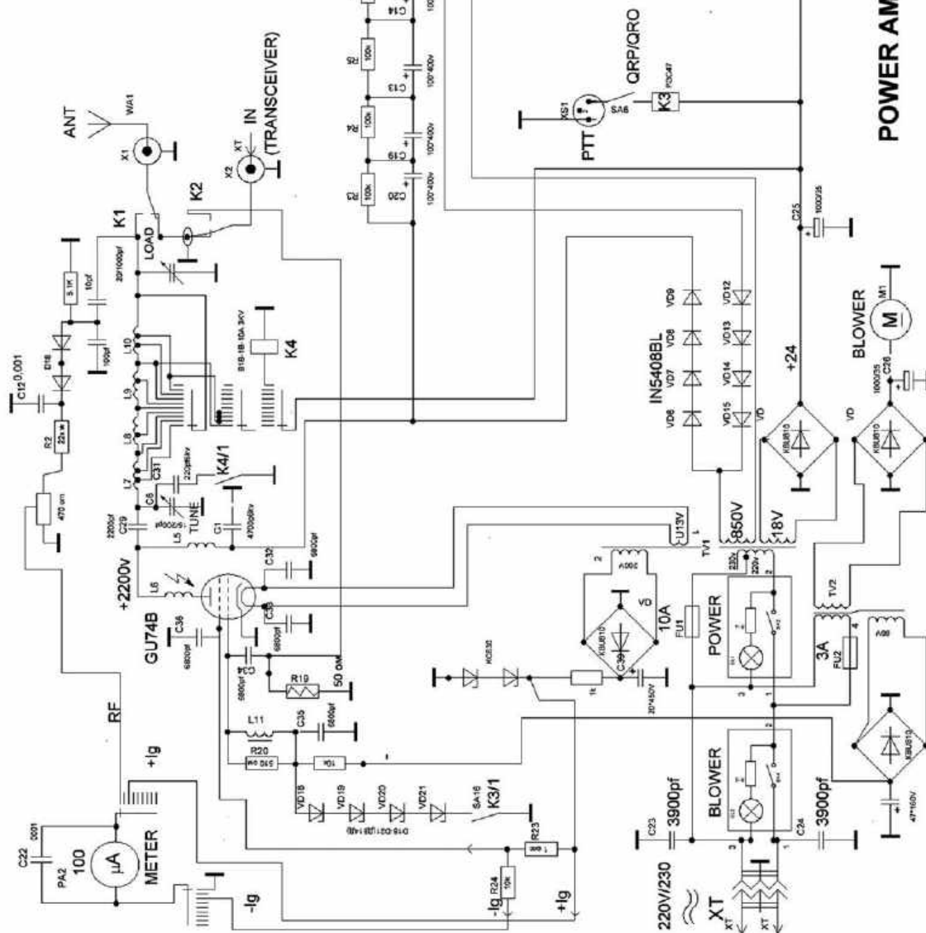
Rys. 2. Schemat lampowego wzmacniacza mocy ZZ-750
