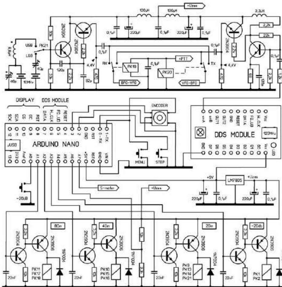
Rys. 5. Schemat układu sterowania Arduino Nano z modulem DDS
