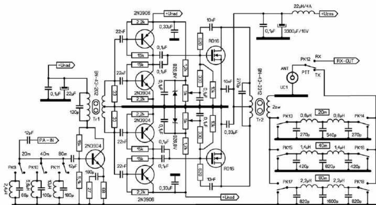
Rys. 4. Schemat wzmacniacza mocy z filtrami wejściowymi i filtrami dolnoprzepustowymi na wyjściu
