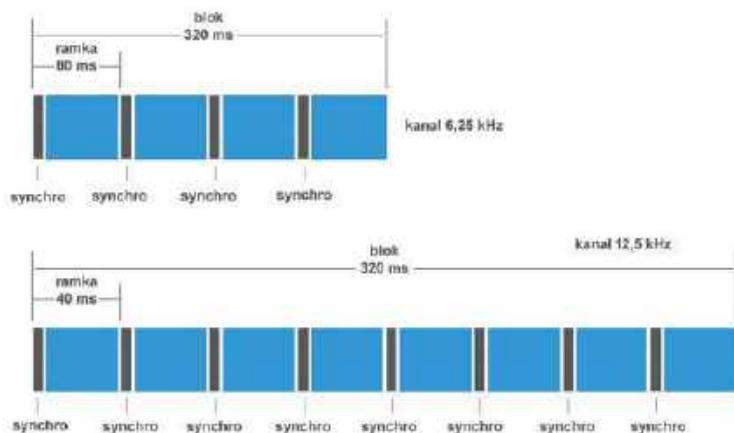
Rys. 3. Bloki danych dla transmisji NXDN w kanale o szerokości 6,25 kHz (u góry) i 12,5 kHz (u dołu)
