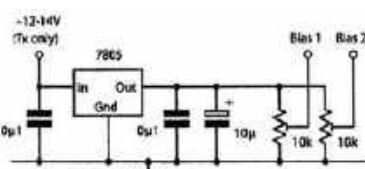
Rys. 2. Schemat układu polaryzacji bramek
