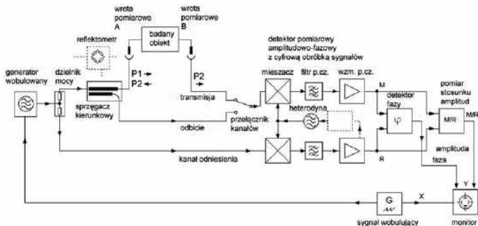
Rys. 4. Uproszczony schemat funkcjonalny analizatora wektorowego
