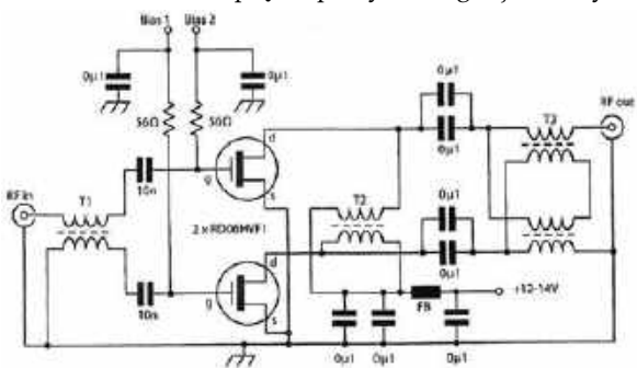
Rys. 1. Schemat przeciwobnego wzmacniacza mocy
