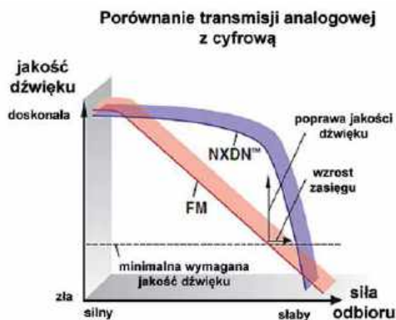
Rys. 2. Zysk w transmisji cyfrowej w porównaniu z analogową
