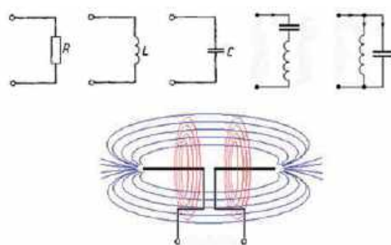
Rys. 3. Przykłady dwójników: podzespoły RLC, obwody rezonansowe i antena
