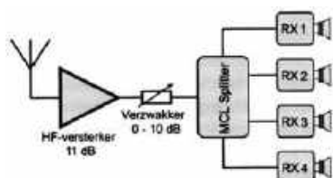
Rys. 4. Schemat blokowy układu pomiarowego
