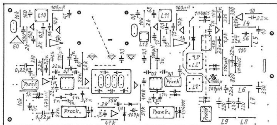
Rys. 3. Rozmieszczenie elementów na płycie
