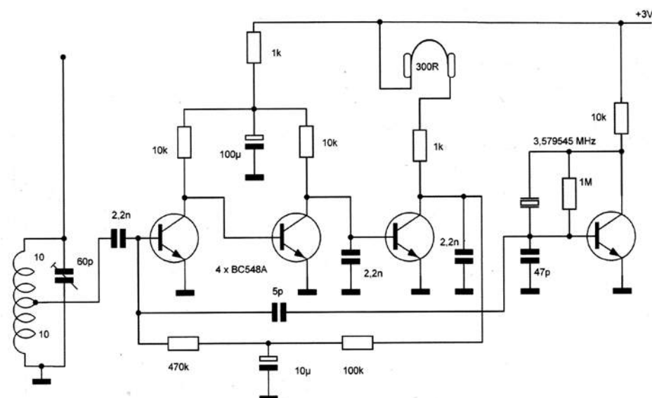
Rys. 4. Schemat odbiornika Fox na 80 m
