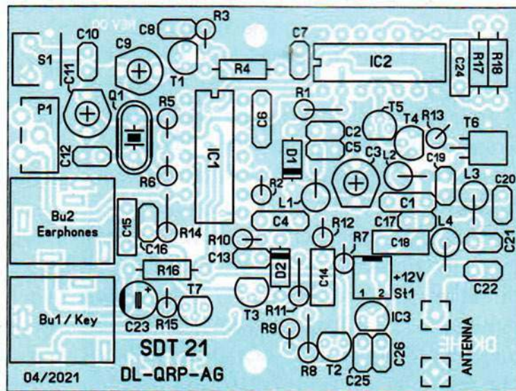
Rys. 6. Rozmieszczenie elementów na płycie SDT21
