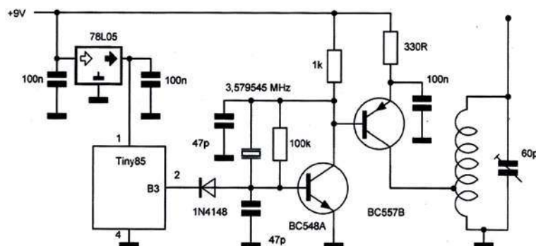
Rys. 3. Schemat nadainika Fox na 80 m
