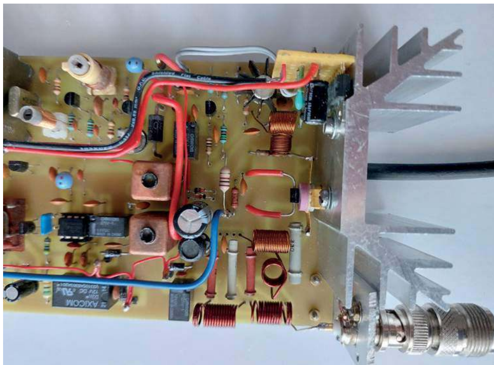
Wnętrze transceivera. W prawym górnym rogu widoczny stopień mocy
