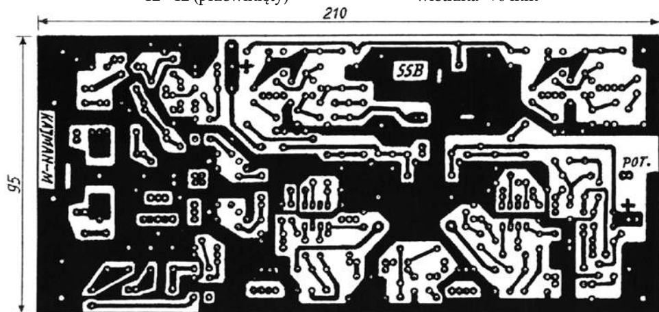
Rys. 2. Szkic jednostronnej płytki drukowanej
