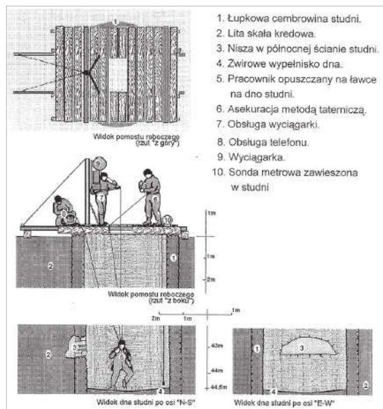
Schematyczne wyobrażenie pomostu roboczego i prowadzenia zjazdów na dno studni podczas badań penetacyjnych 5-8 grudnia 1996 r., rys. Karol E. Natkański.
