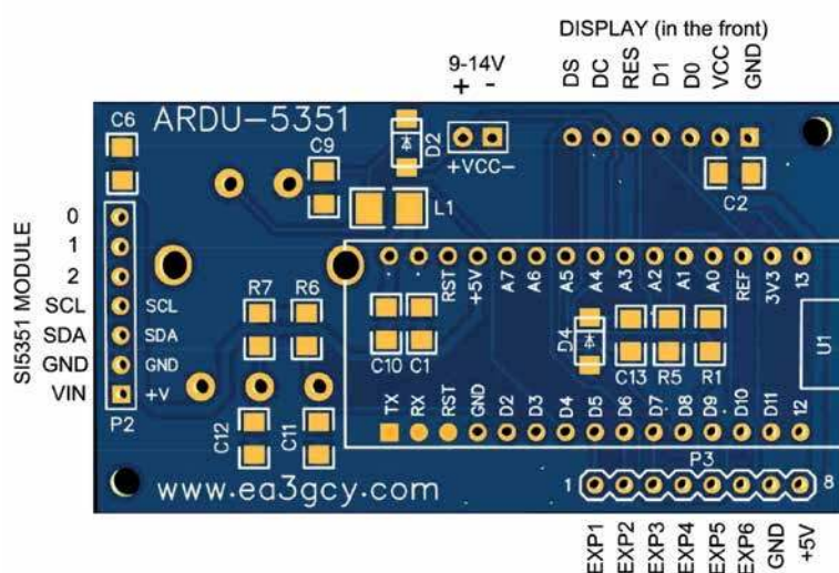
Rys. 3. Rozkład wyprowadzeń modułu SI5351
