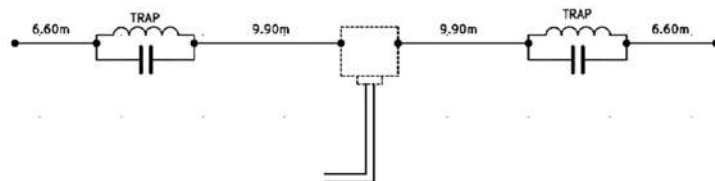
Rys. 1. Schemat anteny W3DZZ wg SQ1GU
