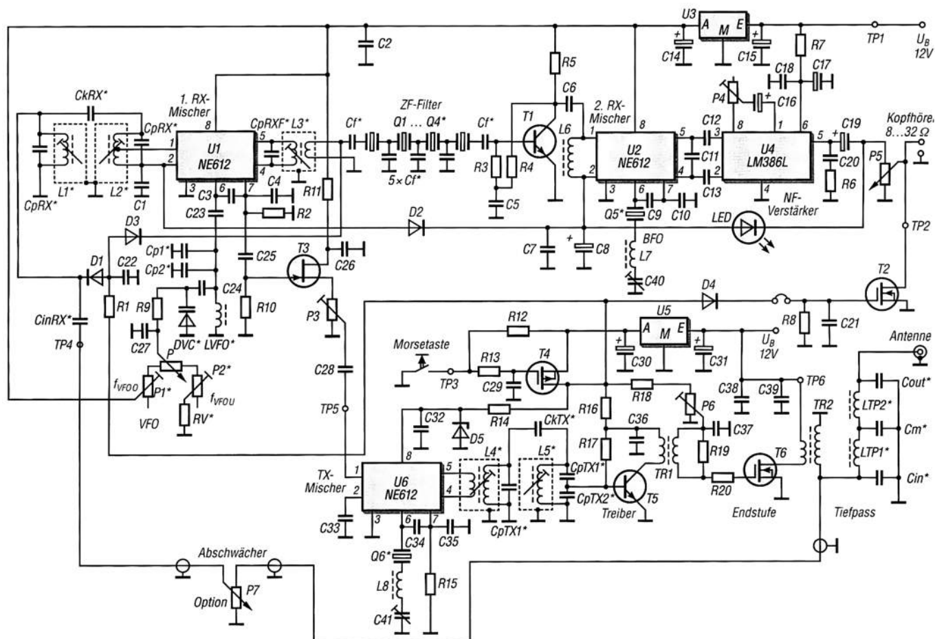
Rys. 4. Schemat ideowy transceivera CW wg DC0DA
