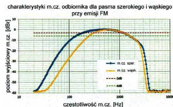
Rys. 8. Wpływ zmian szerokości pasma m.cz. na charakterystykę częstotliwościową
