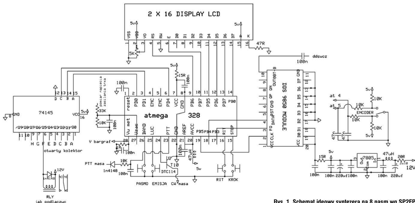
Rys. 1. Schemat ideowy syntezeru na 8 pasm wg SP2FP
