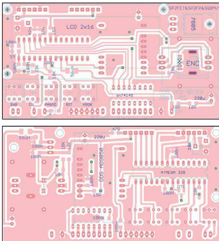
Rys. 2. Dwustronna płytka syntezy DDS wg SP2FP
