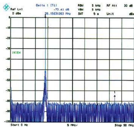
Rys. 9. Widma sygnału nadawanego
