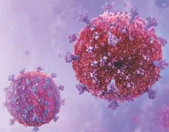
Fot. Corona Borealis
