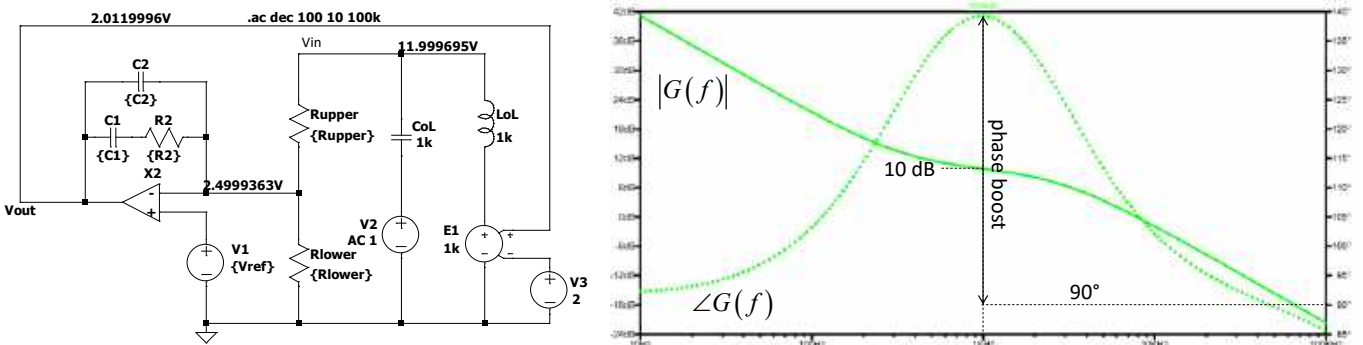
Rysunek 5. Kompensator typu 2 zbudowany na wzmacniaczu operacyjnym oferuje potencjalne doładowanie fazowe do 90°
