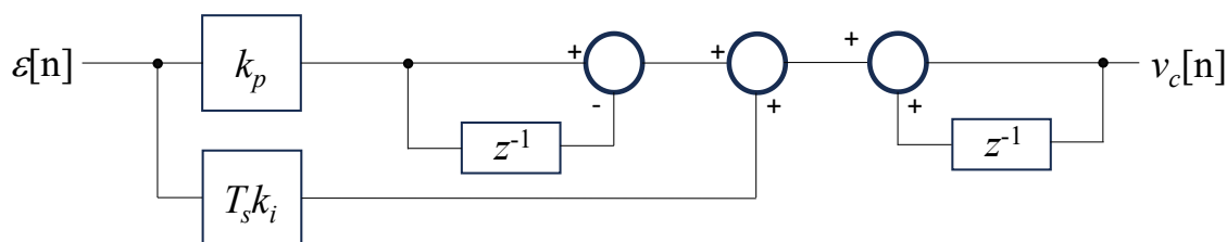
Rysunek 7. Wsteczna transformacja Eulera jest stosowana do transmitancji PI w dziedzinie Laplace'a w celu uzyskania równania różnicowego v_c[n]
