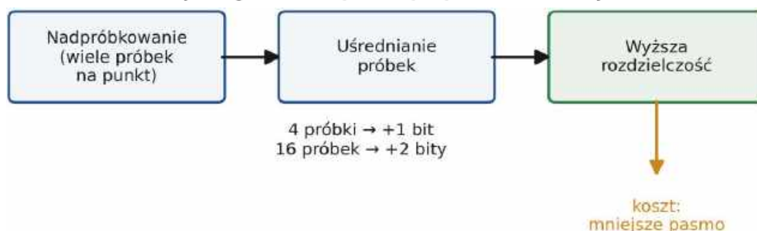
Rysunek 3 Tryb High-Res: nadpróbkowanie i uśrednianie zamieniają nadmiar próbek na dodatkowe bity rozdzielczości – kosztem pasma
