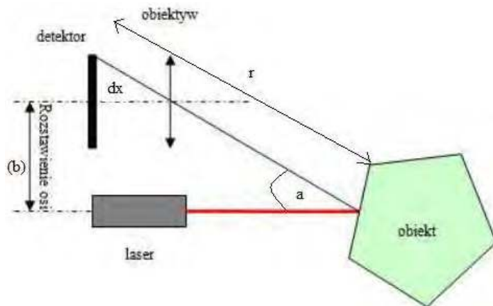
Rysunek 5. Pomiar odległości metodą triangulacji laserowej w oparciu o „Techniki odwzorowania współrzędnych powierzchni 3D – Metoda triangulacji laserowej (ang. laser triangulation)”.
