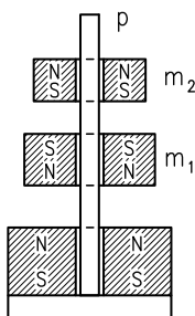
Rys. 11. Układ do badania bezkontaktowego odbicia w układzie magnesów pierścieniowych o masach m_1 , m_2 , prowadzonych wzdłuż pionowego pręta p, pokazany w przekroju osiowym.
