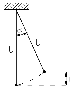
Rys. 6. Schemat do obliczania wysokości h wznesienia kulki po zderzeniu, zwieszonej na nici o długości l , odchylonej o kąt \alpha .
