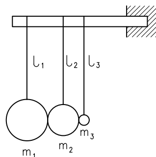
Rys. 12. Układ trzech kulek o masach m_1 , m_2 , m_3 , zawieszonych na niciach o długościach l_1 , l_2 , l_3 , przeznaczonych do uzyskania wielokrotnego wzrostu prędkości po odbiciu ostatniej kulki o masie m_3 . Masy kulek powinny spełniać warunek m_1 \gg m_2 \gg m_3 .
