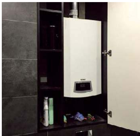
❗ Kocioł z zamkniętą komorą spalania nie czerpie powietrza z pomieszczenia, w którym go zainstalowano. Nie ma więc dokuczliwego efektu wychłodzenia danego wnętrza. TERMET
