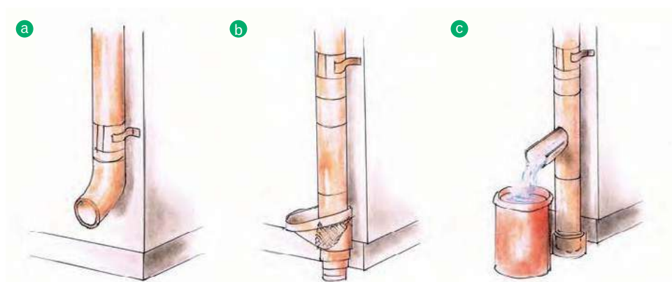
📌 W zależności od tego, gdzie trafia deszczówka, stosuje się różne zakończenia rynien: kolanko kierujące wodę na trawnik (a), lej przy odprowadzeniu do kanalizacji lub studni rozsączającej (b), łapacz deszczówki (c).
