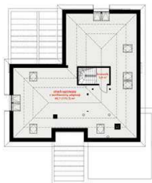
RZUT PODDASZA
