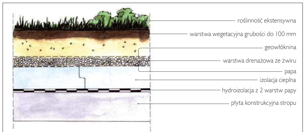
❷ Dach zielony z tradycyjnych materiałów – żwirową warstwą drenującą i stosunkowo grubym podłożem dla roślin – stanowi bardzo duże obciążenie.
