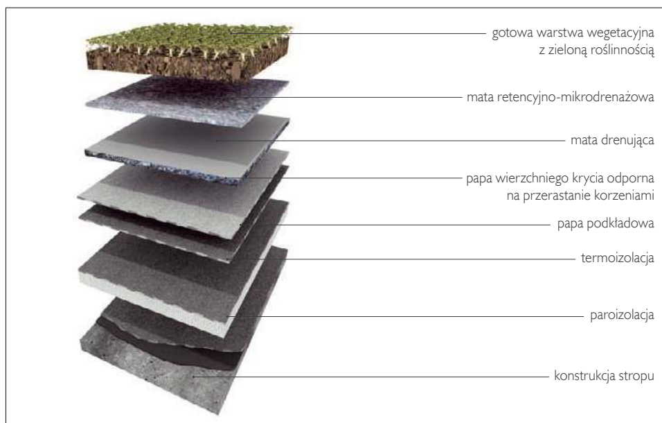
📌 Warstwy systemowego dachu zielonego. Dużym atutem tego rozwiązania jest niewielka grubość i lekkość – poniżej 60 kg/m 2 . ICOPAL
