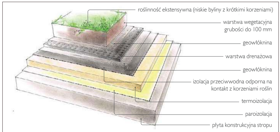
❶ Dach z roślinnością o niewielkich wymaganiach i płytkim systemie korzeniowym.
