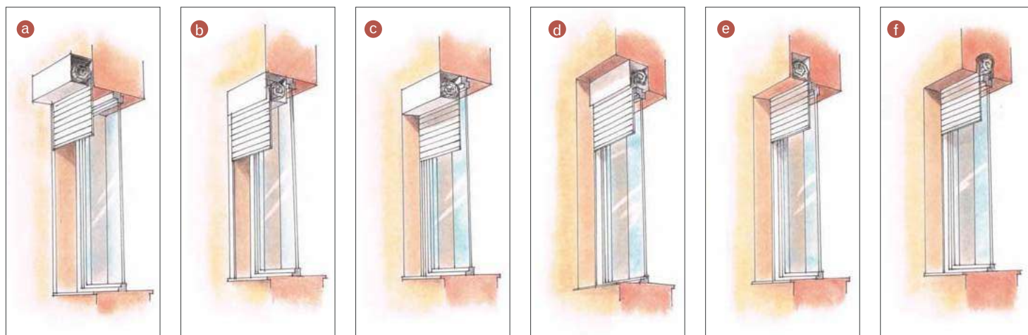
📌 Ze względu na sposób montażu wyróżnia się następujące typy rolet: elewacyjne (a), naokienne prawoskrętnie zwijane (b), naokienne lewoskrętnie zwijane (c), nakładane (d), do zabudowy (e), nadprożowe (f).
