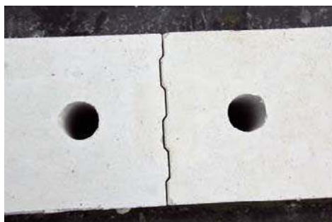
🔧 Elementy łączone na pióro i wpust nie wymagają stosowania spoiny pionowej. J. WERNER
