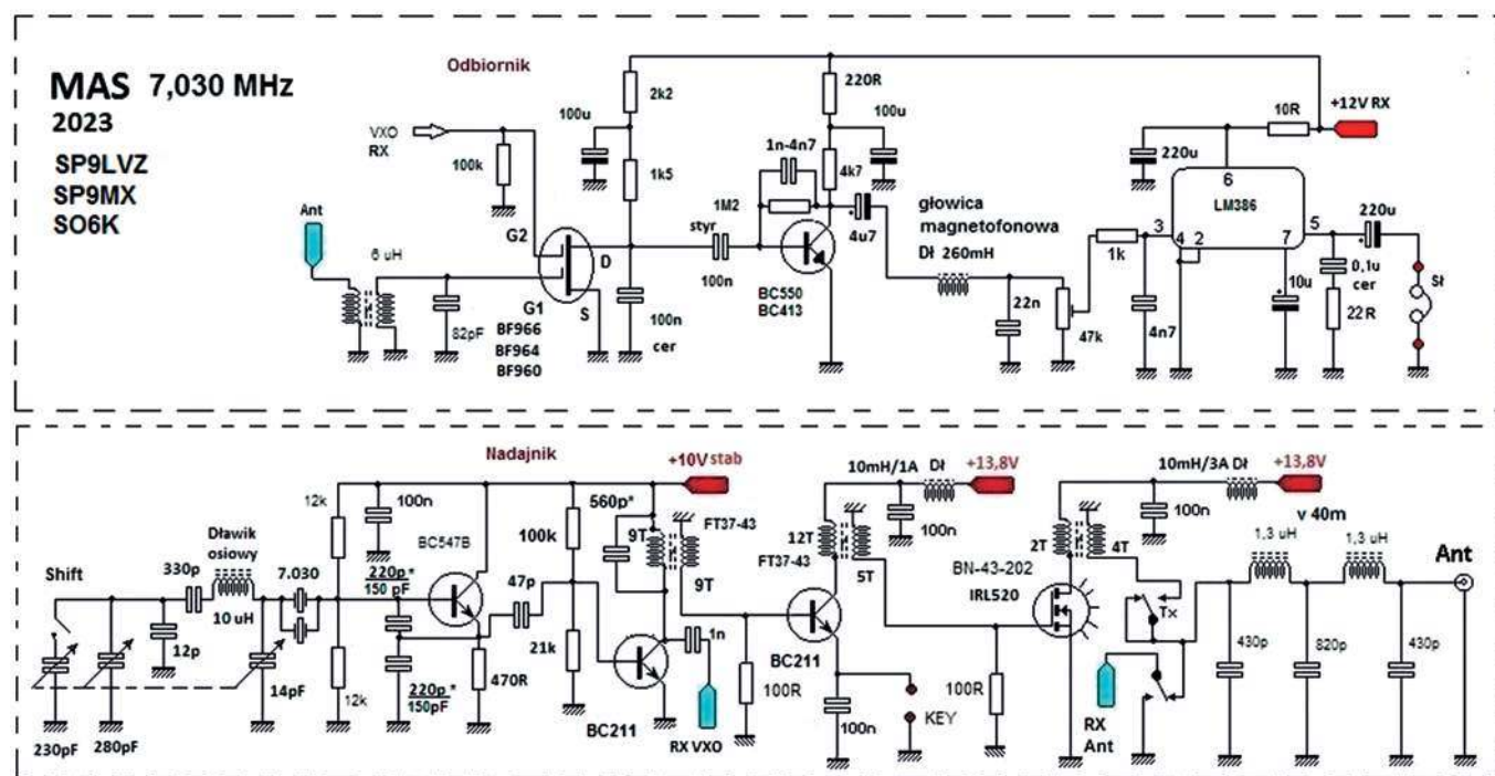
Rys. 1. Schemat ideowy transceiwera na pasmo 7 MHz
