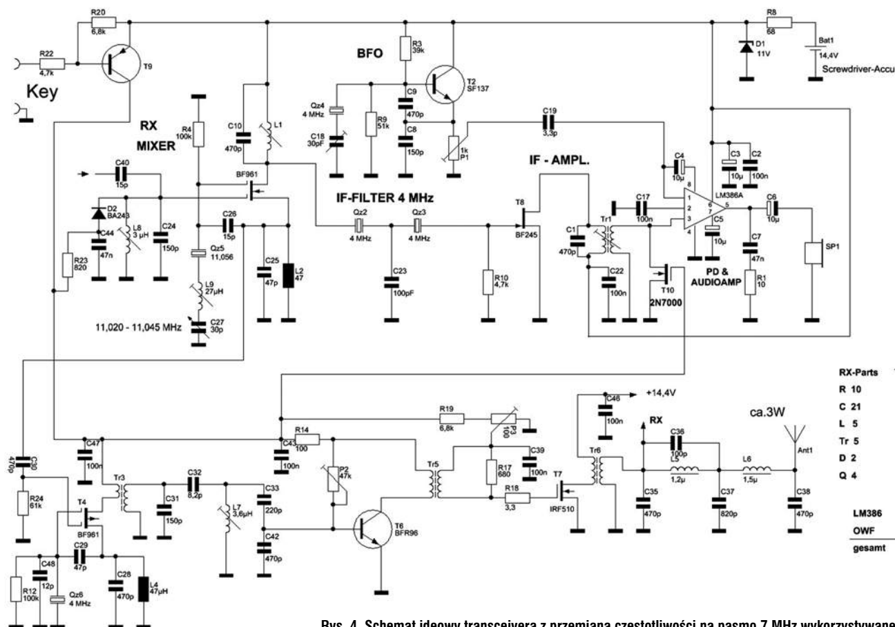
Rys. 4. Schemat ideowy transceivera z przemianą częstotliwości na pasmo 7 MHz wykorzystanego przez DL6GCG
