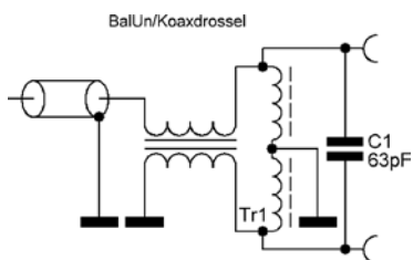
Rys. 3. Schemat ideowy baluna
