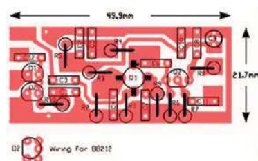
Rys. 10. Płytką drukowaną wzmacniacza z rozmieszczeniem elementów
