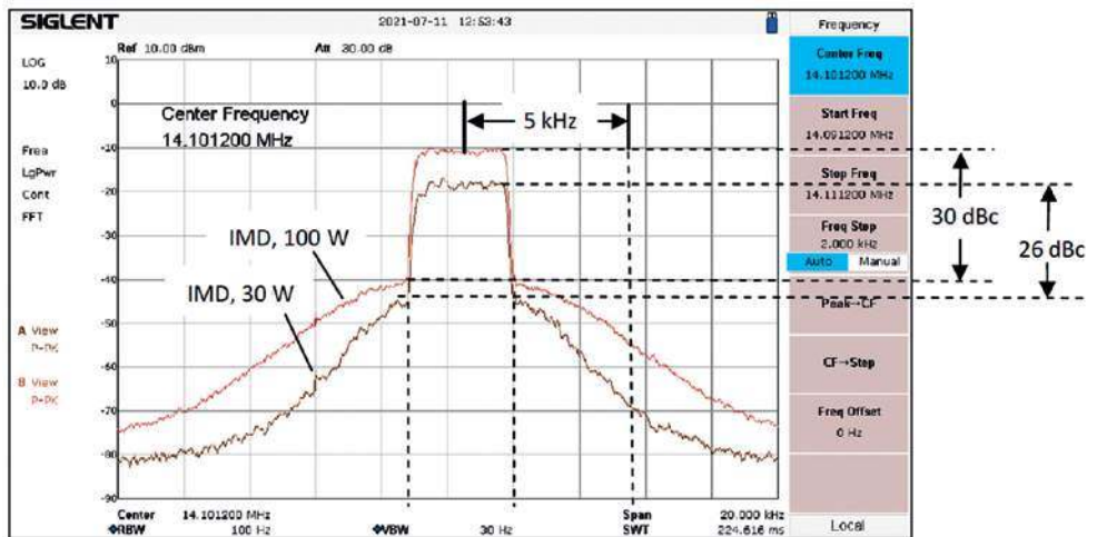
Rys. 5. Pomiar dla nadajnika wyższej klasy (IMD3 – 42 dBc)
