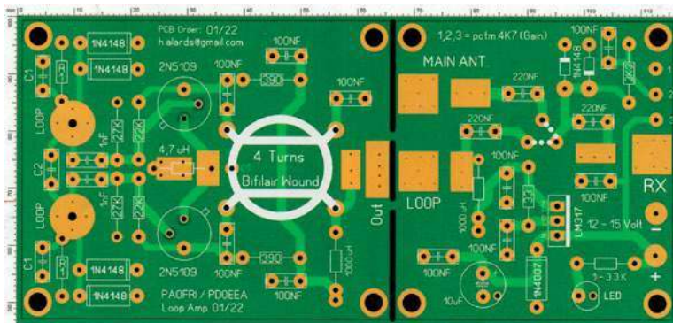
Rys. 8. Płytki montażowe PCB wzmacniacza z rozmieszczeniem elementów
