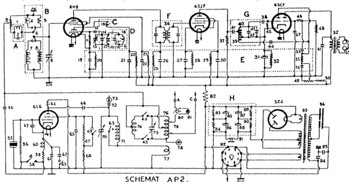
Schemat radiostacji AP-2
