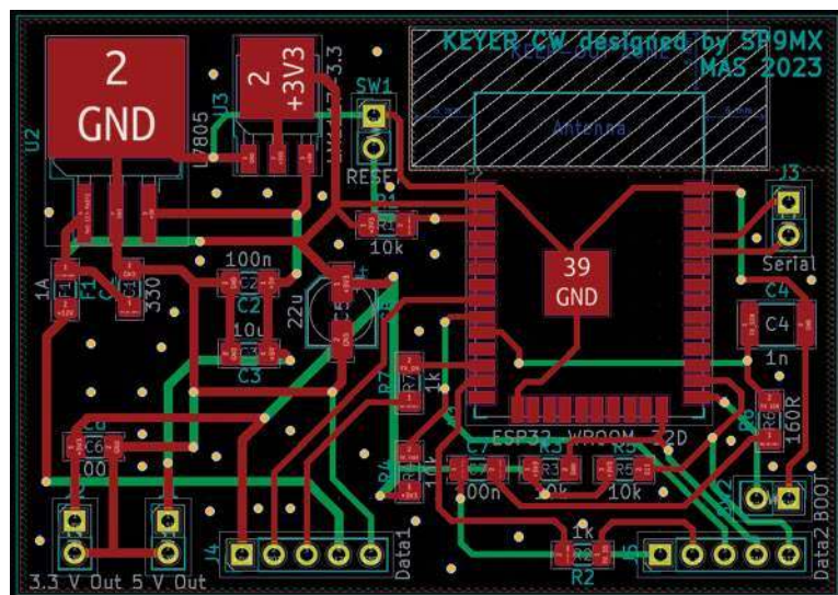
Rys. 2. Rozmieszczenie ścieżek i elementów na płycie drukowanej
