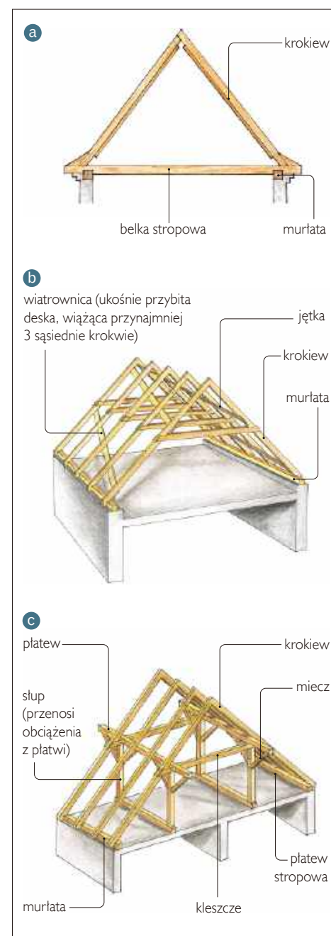
🔧 Tradycyjna więzba dachowa: krokwiowa (a), krokwiowo-jętkowa (b), płatwiowo-kleszczowa (c).
