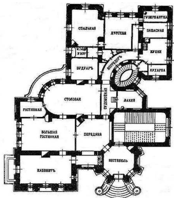
План помешкання Городецького в «Будинку з химерами»
