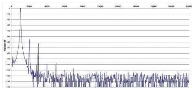
Rys. 2a. Zniekształcenia harmoniczne, tryb triodowy.
