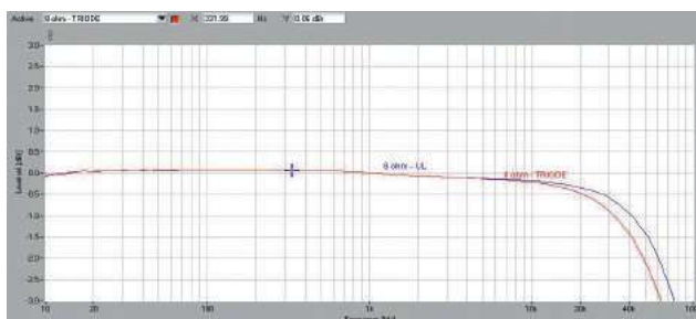
Rys. 1b. Pasma przenoszenia, tryb triodowy i UL, 8 \Omega .
