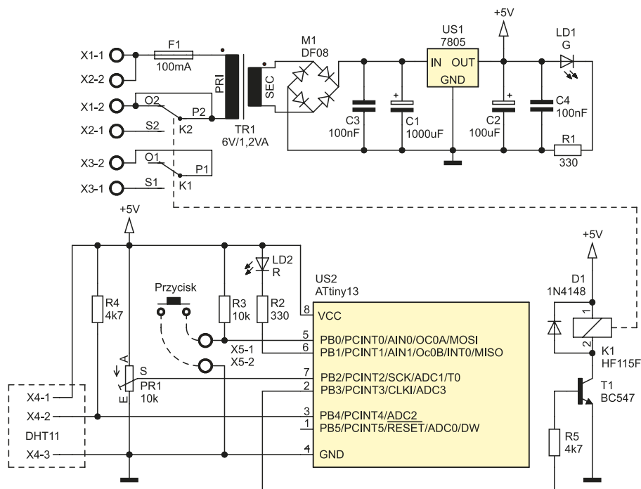
1. Schemat ideowy sterownika wentylatora
