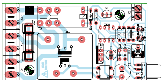
2. Schemat montażowy sterownika wentylatora
