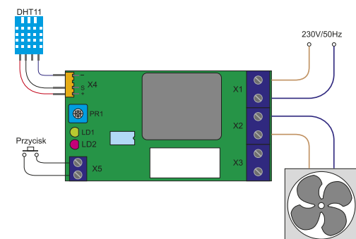
3. Dołączenie sterownika do sieci energetycznej
