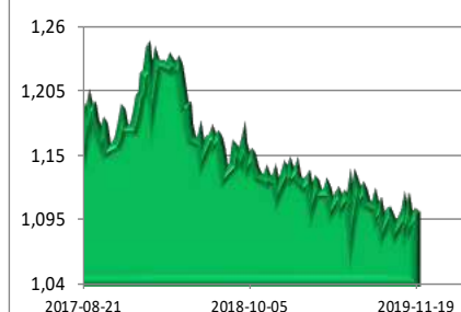
GBP/USD
