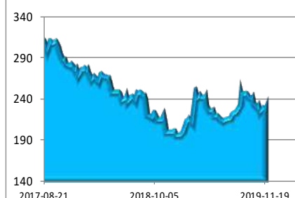
DJIA
