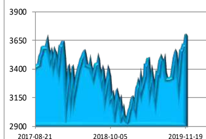
EUR/USD
