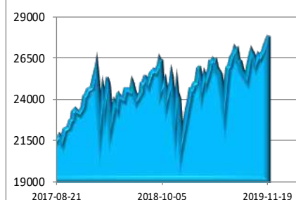
EURO STOXX 50
