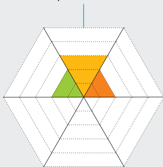
Teoria pamięci, świadomości i temporalności (MCTT)
