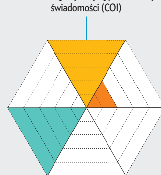
Teoria integracji międzypoziomowej świadomości (COI)
