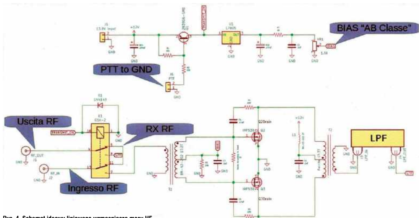
Rys. 4. Schemat ideowy liniowego wzmacniacza mocy HF
