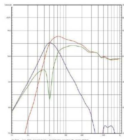
Rys. 4. SourcePoint 8. Charakterystyki źródeł sekcji niskotonowej (poniżej 1 kHz, pomiar w polu bliskim) – głośnik, bas-refleks, wypadkowa.
