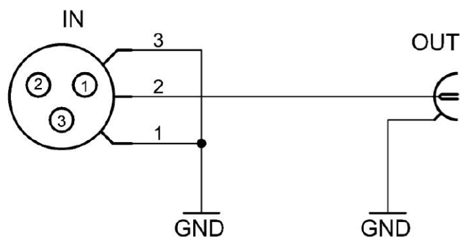
Rysunek 1. Najprostsze podłączenia wejścia zbalansowanego
