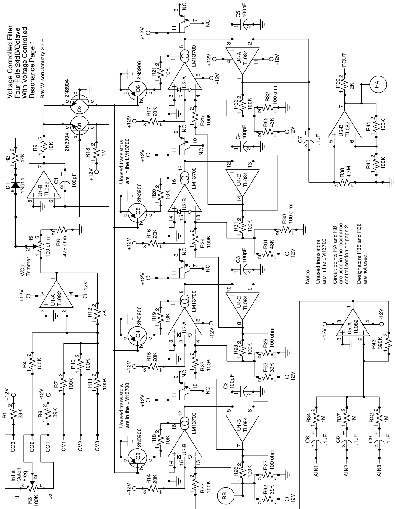
Rysunek 1. Schemat filtra sterowanego napięciem – sekcja główna
