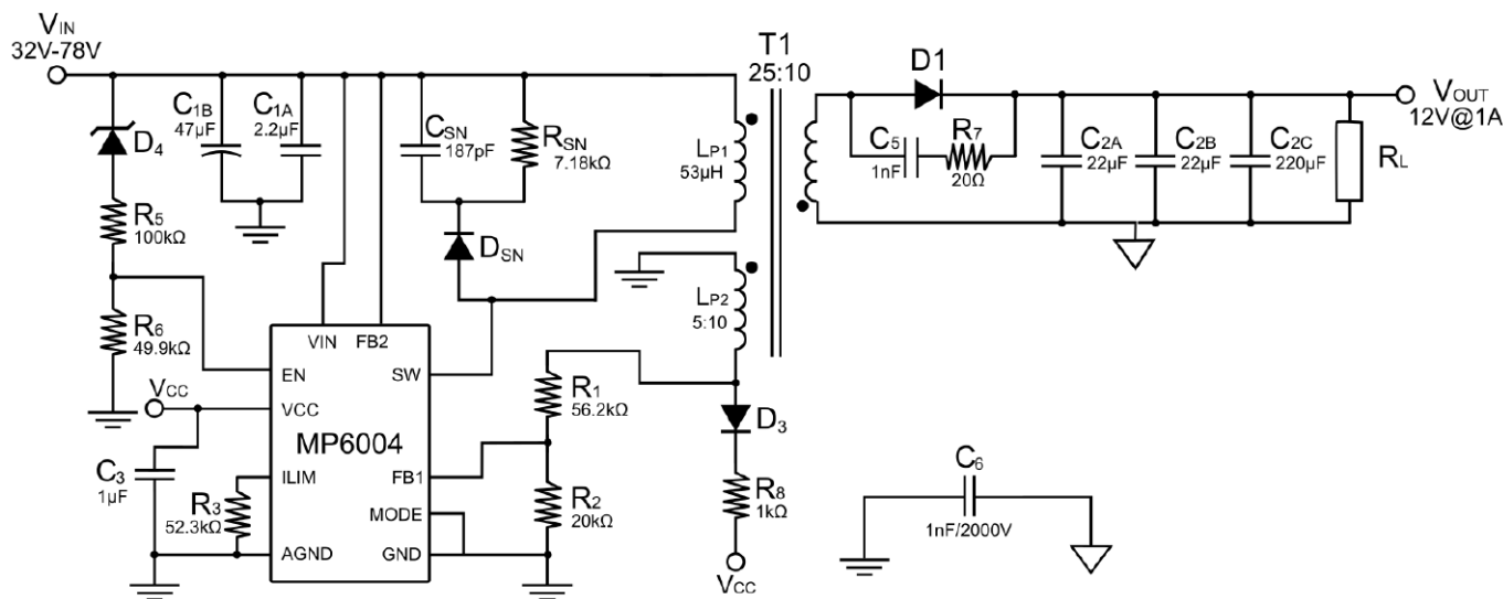
Rysunek 6. Kompletny schemat przetwornicy flyback 12 V/1 A z kontrolerem MP6004 (primary-side regulation). Źródło: T. Hudson, M. Ametller, AN0067 Rev. 1.0, © 2022 Monolithic Power Systems – reprodukowano za uprzejmą zgodą Autorów
