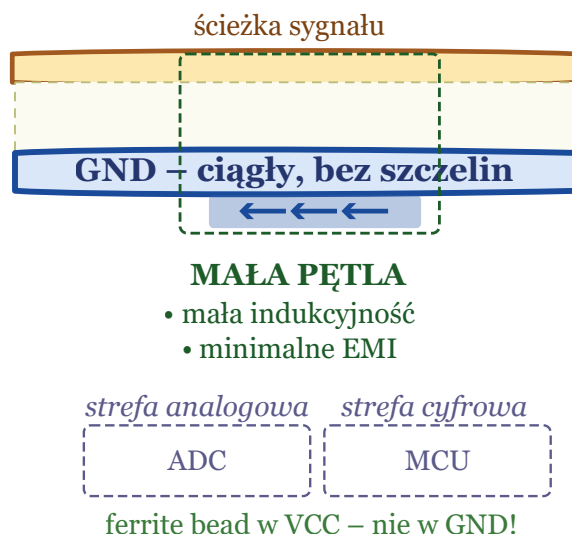
Rysunek 3. Dzielona płaszczyzna vs ciągła płaszczyzna GND – ścieżki prądów powrotnych i separacja funkcjonalna. Przy podziale płaszczyzny masy prąd powrotny musi obejść szczelinę przez mostek, tworząc pętlę indukcyjną. Przy ciągłej płaszczyźnie GND prąd wraca bezpośrednio pod ścieżką. Separację domen osiągamy przez rozmieszczenie bloków nad płaszczyzną, nie przez jej cięcie (na podstawie: Hartley 2019; TI SLYT512; Altium „How to Properly Ground ADCs”)
