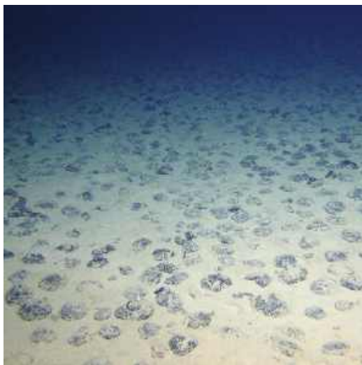
5. Konkrecje na dnie strefy Clarion-Clipperton Pacyfiku
