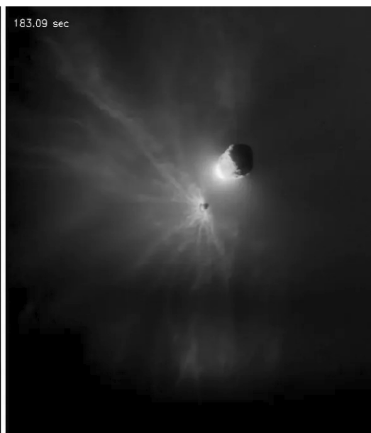
1. Zdjęcia wykonane kilka minut po impakcie w Dimorfosa, przedstawiające wyrzut powstały w wyniku kolizji © NASA
