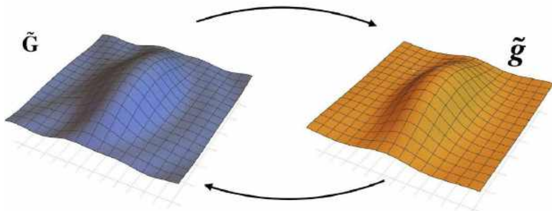
3. Schematyczna i matematyczna reprezentacja entropijnego działania kwantowej grawitacji
