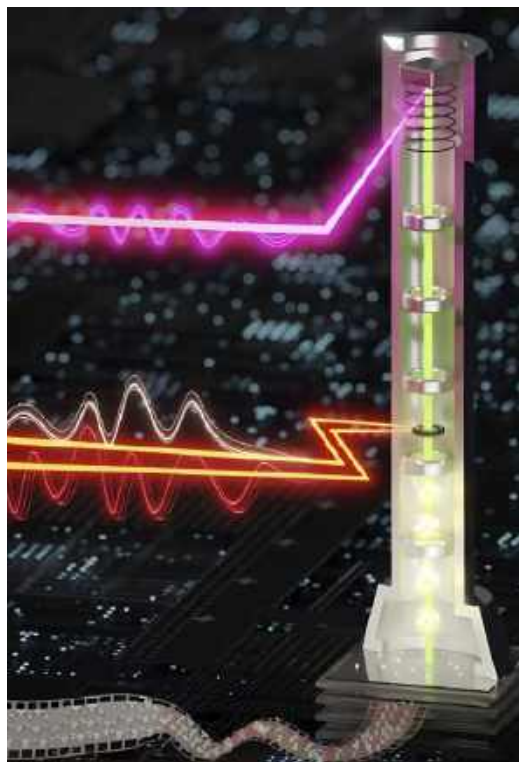
5. Ilustracja działania atomomikroskopu © University of Arizona
