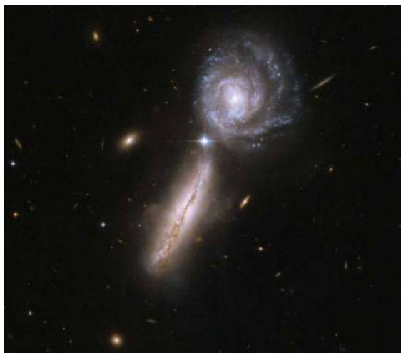
Te dwie bardzo zasobne w gaz galaktyki spiralne znajdują się we wstępnej fazie kolizji. Noszą nazwę UGC 9618, a w katalogu Arpa – Arp 302.
