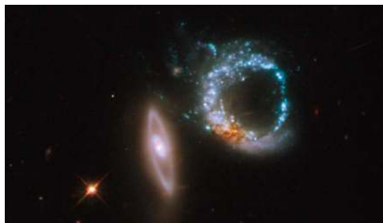
Para oddziałujących ze sobą galaktyk uchwycona przez teleskop Hubble'a. W katalogu Arpa numer 147
