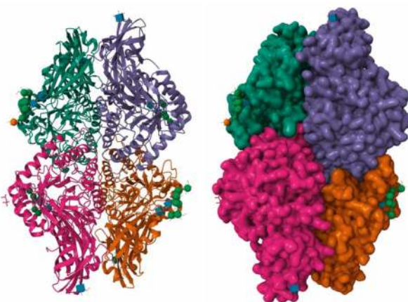
\beta -glukuronidaza składa się z czterech identycznych podjednostek.
