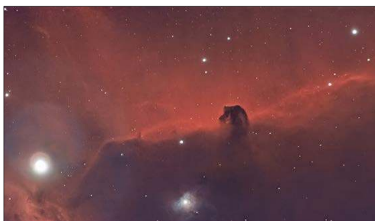
Zdjęcie mgławicy Koński Łeb (IC 434) wykonane teleskopem Seestar 50 w dniu 31.10.2025 w centrum Dębicy. fot. Bartłomiej Janowski
