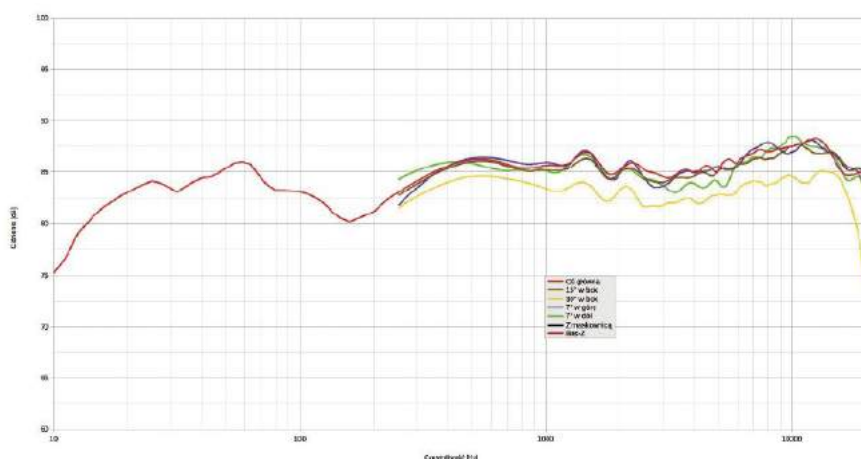
Rys. 1 Charakterystyka przetwarzania w całym paśmie, na różnych osiach (w trybie Narrow).
