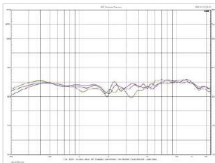
Rys. 6b. Charakterystyka w zakresie średnio-wysokotonowym, na różnych osiach, w płaszczyźnie pionowej, w trybie Wide.
