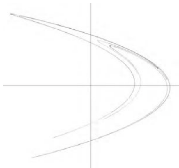
Rys. 11. Wykres atraktora Henona. Źródło obrazka: https://pl.wikipedia.org/wiki/Uk%C5%82ad_Henona#/media/Plik:Henon_attractor.png
