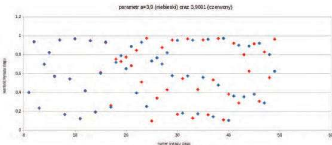
Rys. 5. Zestawienie rozkładu punktów otrzymanych z równania logistycznego dla stałych a=3,9 i a=3,9001 .
