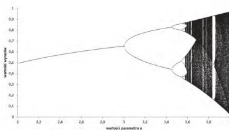
Rys. 6. Zestawienie rozkładu punktów generowanych dla równania logistycznego z wartościami stałej a w przedziale \langle 2,4 \rangle .
