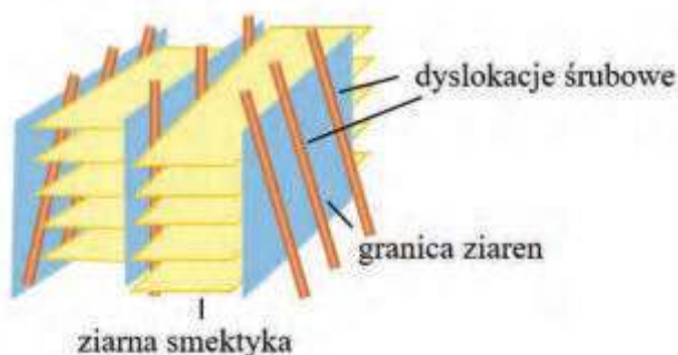
Rysunek 2. Schemat struktury fazy TGB-A. Ziarna smektyka nie muszą mieć struktury smektyka A. Obserwowano również fazy TGB, którym ziarnom przypisano strukturę pochylonego smektyka C (TGB-C), a nawet chiralnego smektyka C.
