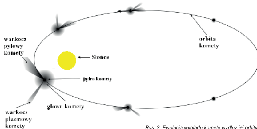
Rys. 3. Evolucja wyglądu komety wzdłuż jej orbity.
