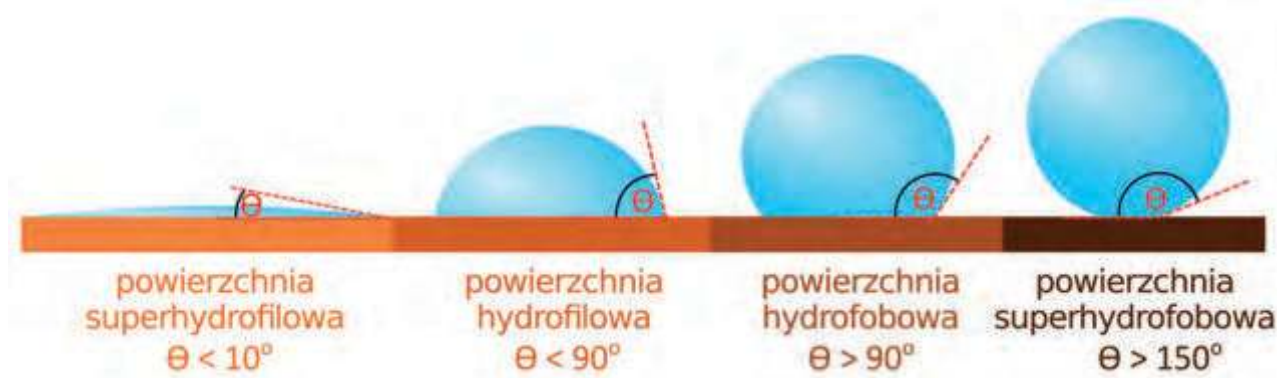
Rys. 6. Kąty zwilżania dla kropli wody umieszczonej na podłożach o odmiennych właściwościach.
