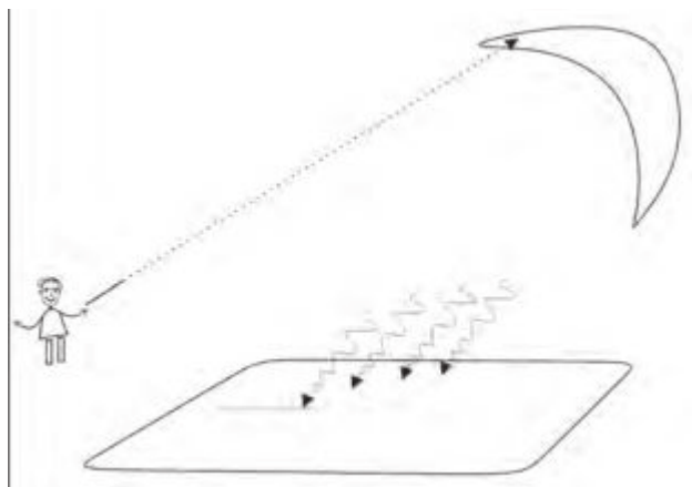
Rys. 3. „Zajączek” na Księżycu. Struga światła (np. z lasera) przeciągnięta przez Księżyc bez trudu przekracza prędkość światła sugerując, że plamka świetlna biegnąca przez Księżyc ma wątpliwą fizyczność. Rzeczywiście na dole rysunku przedstawiona jest powierzchnia Księżyca do której dobiegają fotony. Oczywiście „zajączka” tworzą w każdym miejscu inne fotony (których prędkość wynosi „c”). Fizyczna jest prędkość fotonów a nie biegnącego zajączka.
