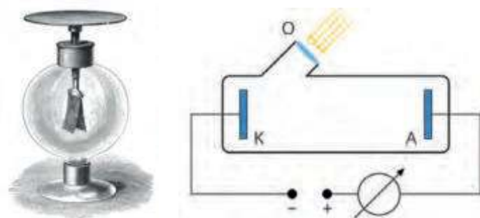
Rysunek 1. Jeden z pierwszych zestawów do demonstracji efektu fotoelektrycznego. Schemat układu doświadczalnego do badania zjawiska fotoelektrycznego
