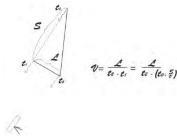
Rys. 4. „Nadświatłny” ruch rzutu dżetu na sferze niebieskiej. Mierzona prędkość to wynik dzielenia drogi w kierunku prostopadłym do linii widzenia (na sferze niebieskiej) przez różnicę czasów t_2 - t_1 , dotarcia do teleskopu fotonów z końców widocznego na sferze dżetu. Oczywiście ta różnica czasów jest równa różnicy czasów zaznaczonych na rysunku. Różnica czasów jest oczywiście mniejsza od L/c i przy dużej (podświetlonej) prędkości dżetu, prędkość rzutu dżetu na sferze niebieskiej bywa większa od prędkości światła. Sytuacja jest więc dość podobna do przedstawionej na Rys. 3. ruchu „zajączka”
