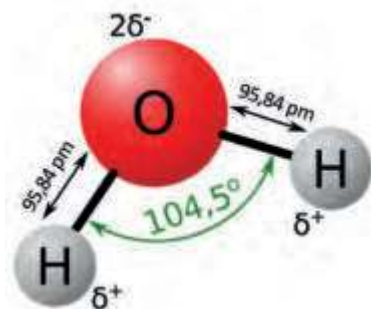
Rys. 1. Uproszczony model cząsteczki wody.
