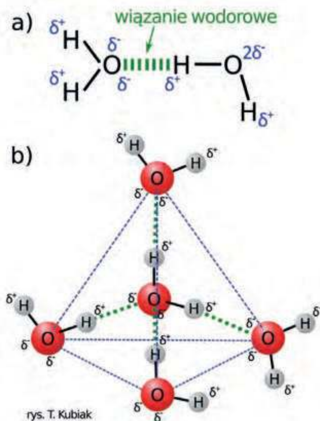
Rys.5 a) Wiązanie wodorowe pomiędzy dwoma molekułami H_2O ; b) cząsteczka H_2O może łączyć się wiązaniami wodorowymi z czterema sąsiednimi, tworząc układ tetraedyczny.
