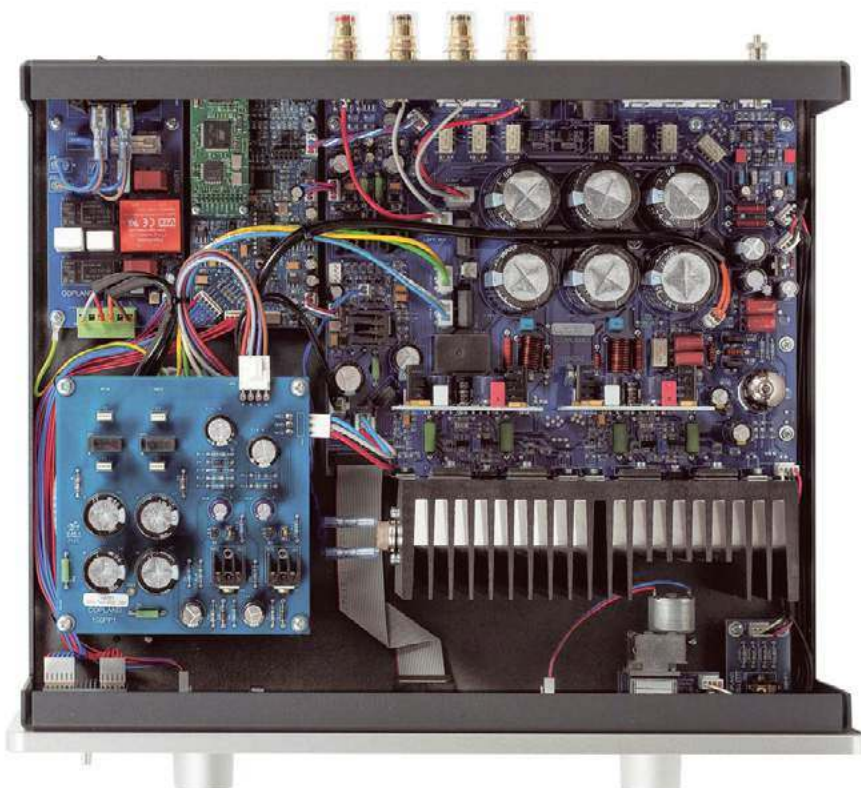
Wnętrze CSA 150 łączy różne techniki: tranzystorową i lampową, analogową i cyfrową.
