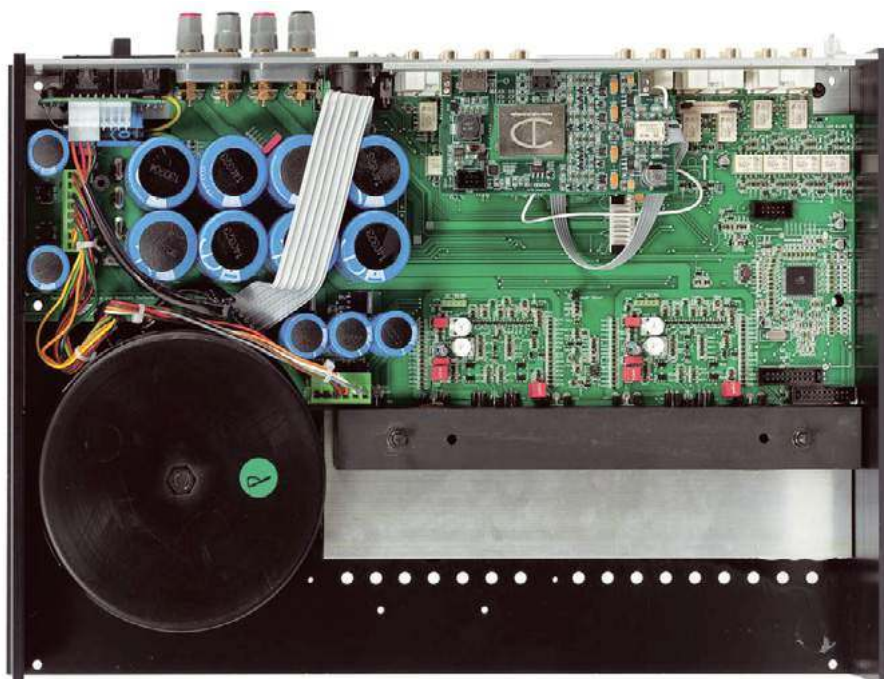
Densen od wielu lat wciska liniowe końcówki mocy w bardzo niskie obudowy – wymaga to zastosowania płaskiego radiatora (i transformatora).
