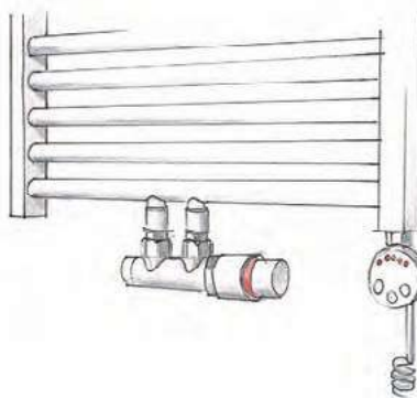
❷ Rys. 2 Podłączenie centralne dolne, tzw. D50. Sprawdzamy po której stronie producent dopuszcza montaż grzałki.
