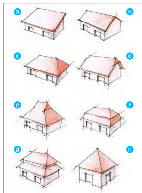
📌 Rodzaje dachów spadzistych: jednospadowy (a), dwuspadowy (b), czterospadowy (c), naczółkowy (d), półszczytowy (e), mansardowy (f), polski (g), namiotowy (h).
