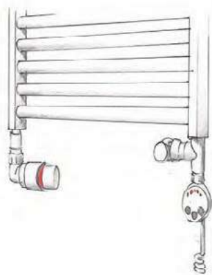
❶ Rys. 1 Typowa drabinka o symetrycznym kształcie ma 2 przyłącza u dołu. Najczęściej grzałkę podłącza się poprzez dodatkowy trójnik założony na powrocie.
