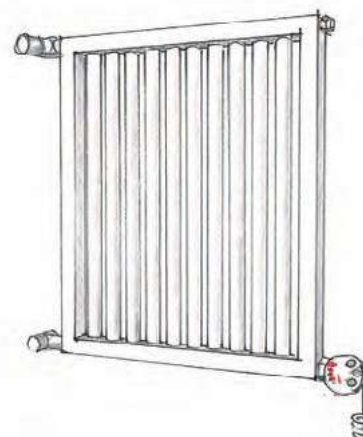
❺ Rys. 5 Podłączenie poziome grzałki dopuszczalne jest sporadycznie i tylko przy pionowym ustawieniu szczebelków.
