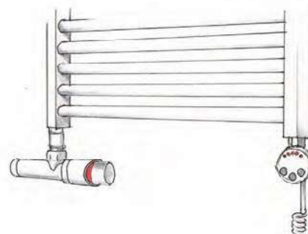
❸ Rys. 3 Podłączenie dolne przez specjalny zawór rurowy. Zasilanie i powrót zajmują wówczas tylko jeden króciec grzejnika.
