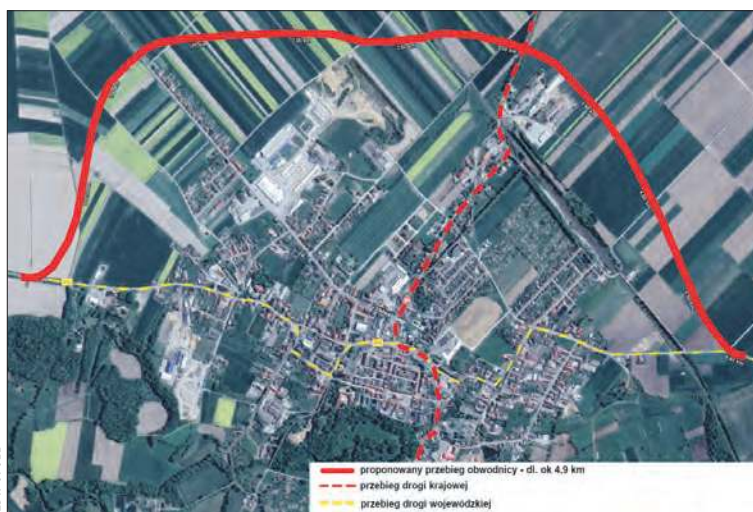
Wstępny projekt przebiegu obwodnicy Głogówka
