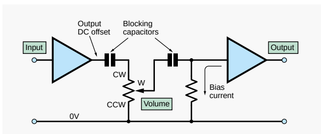
Rysunek 9. Usuwanie składowej stałej sygnału za pomocą kondensatorów sprzęgających
