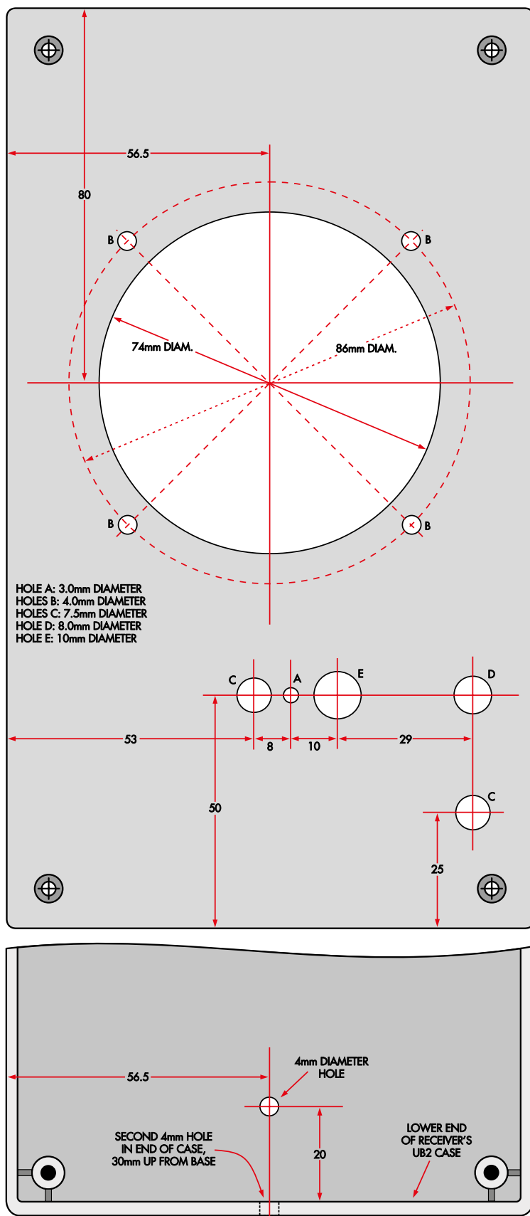
Rysunki 12 i 13. Wykonanie otworów w pokrywie odbiornika (górny rysunek) jest najbardziej pracochłonnym etapem projektu. Wymaga wykonania jednego dużego otworu pod głośnik za pomocą otwornicy oraz sześciu mniejszych otworów. Na dolnym rysunku pokazano położenie dwóch otworów, przez które przechodzi opaska zaciskowa mocująca baterię 9 V
