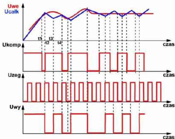
Graficzne wyjaśnienie działania modulatora delta (© 2018 Jos Verstraten)
