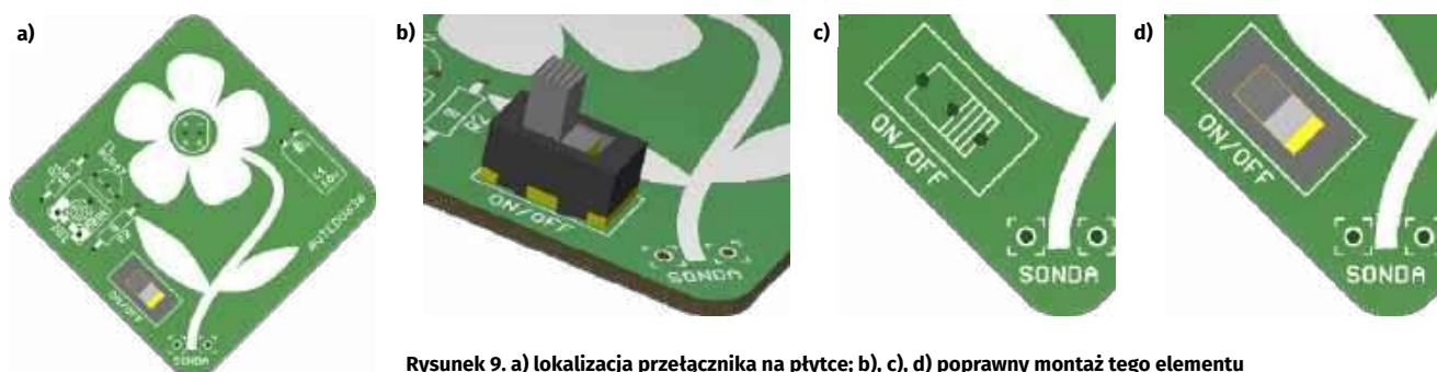
Rysunek 9. a) lokalizacja przełącznika na płytce; b), c), d) poprawny montaż tego elementu
