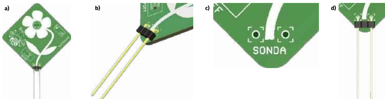
Rysunek 10. a) lokalizacja elementu na płytce; b), c) i d) poprawny montaż tego elementu
