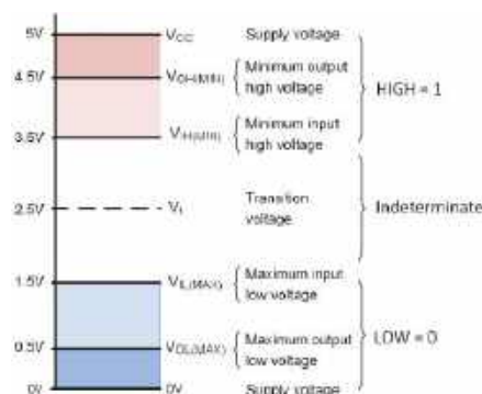
Rysunek 10.6. Standardowe poziomy logiczne dla układów z serii HC
