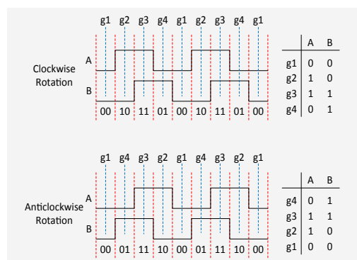
Rysunek 4. Do określenia kierunku obrotów służy sygnał wyprzedzający
