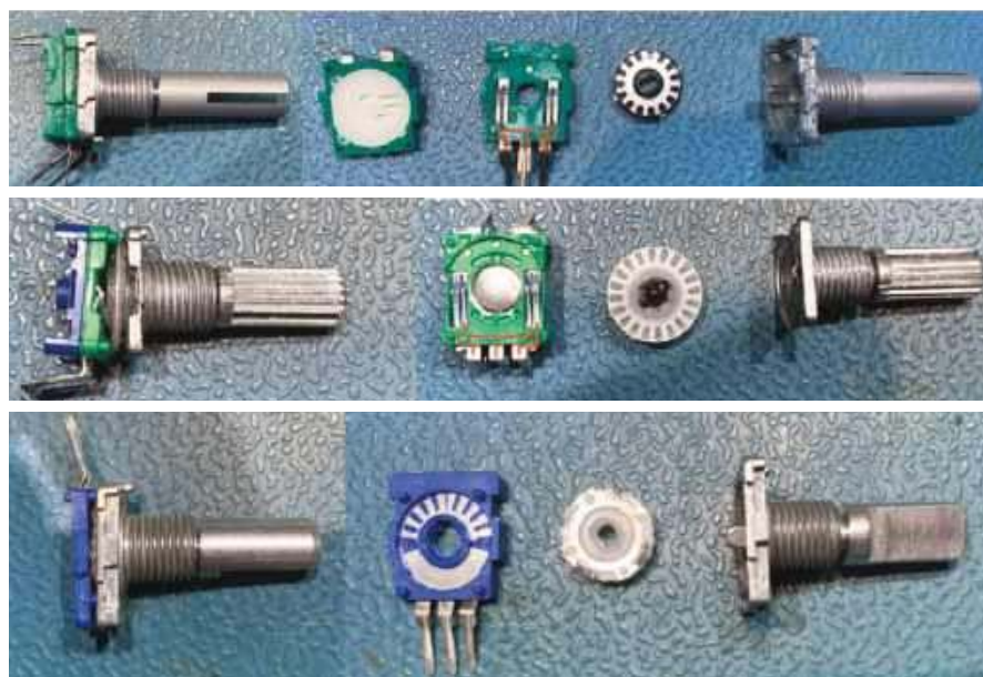
Rysunek 5. Enkodery o liczbie kliknięć 30 (u góry), 20 (w środku) i 20 (u dołu). Zdjęcie: Joe Farr
