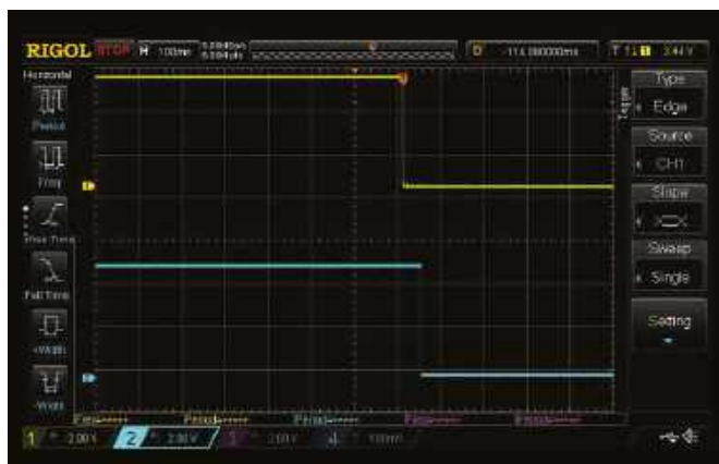
Rysunek 7. Enkoder o 30 kliknięciach. Z lewej: obrót pokrętki o jeden klik w prawo, po prawej: obrót o kolejny klik w prawo
