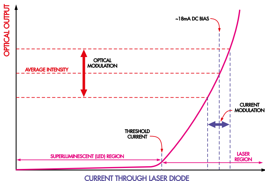
Rysunek 4. Moc optyczna lasera w funkcji prądu wejściowego. Diody laserowe nie emitują promieniowania laserowego, dopóki nie popłynie przez nie wystarczająco duży prąd. Dlatego podczas modulowania mocy lasera konieczne jest ustawienie minimalnego prądu polaryzacji
