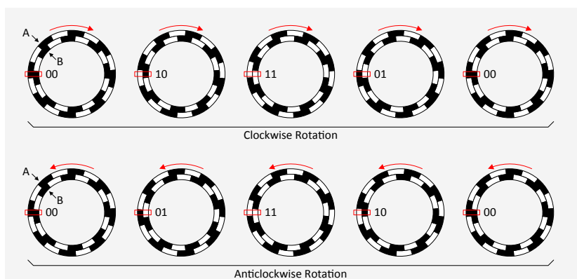
Rysunek 3. Schemat działania obrotowego enkodera kwadraturowego
