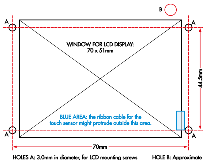
Rysunek 12 (po lewej). Do zamontowania wyświetlacza LCD o przekątnej 2,8 cala, a wraz z nim modułu sterującego-zasilającego, wymagane jest wykonanie dużego prostokątnego wycięcia oraz czterech niewielkich otworów montażowych. Może być również konieczne wykonanie dodatkowego otworu dla odbiornika podczerwieni, umożliwiającego odbiór sygnałów z pilota z zewnątrz obudowy, takiego jak otwór oznaczony literą „B”
