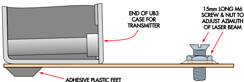
Rysunek 9. Przyklejenie nakrętki do podstawy i wkręcenie w nią śruby pozwala na łatwą regulację kąta nachylenia obudowy względem podłoża w niewielkich krokach, co umożliwia precyzyjne ustawienie wiązki lasera.
