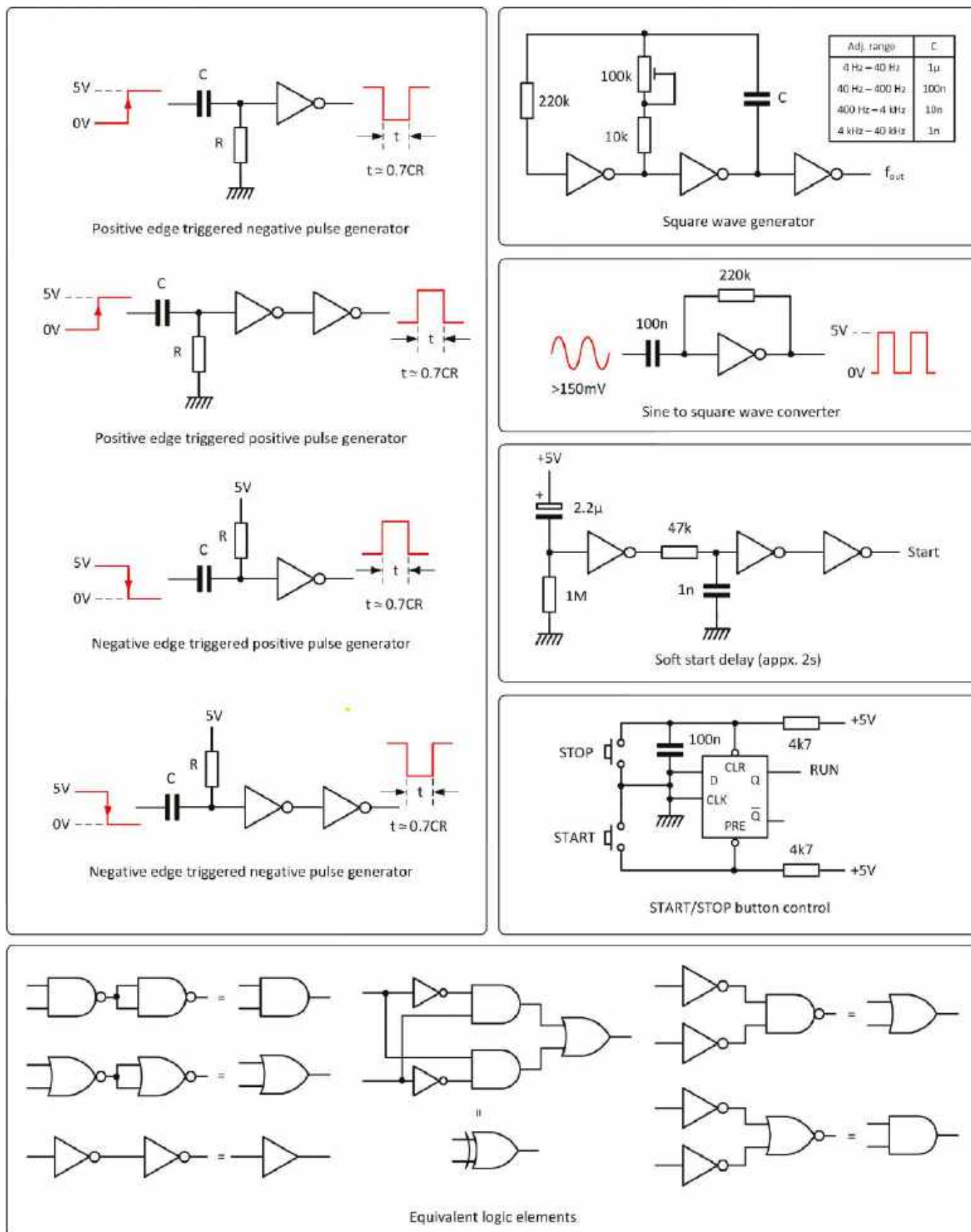
Rysunek 10.15. Trochę przydatnych rozwiązań układowych opartych na „klasycznej logice”
