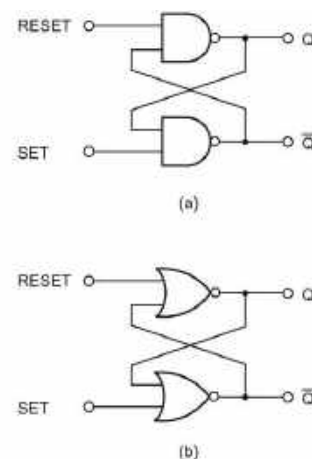
Rysunek 10.4. Użycie sprzężonych na krzyż bramek logicznych NAND i NOR do realizacji bistabilnych przerzutników R-S
