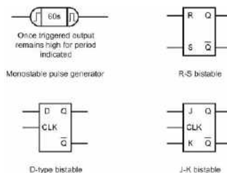
Rysunek 10.3. Symbole przerzutników monostabilnych i bistabilnych
