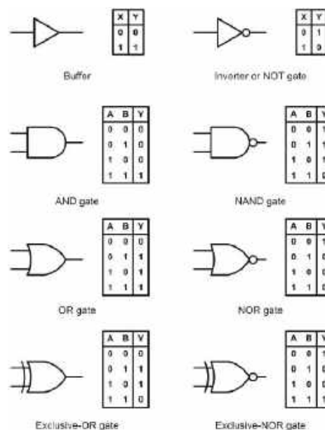
Rysunek 10.2. Symbole podstawowych elementów logicznych wraz z ich tablicami prawdy
