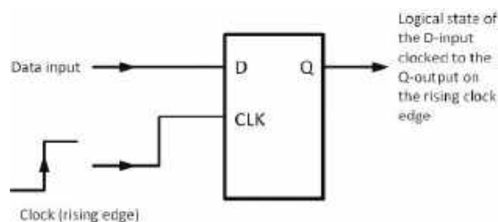
Rysunek 10.5. Taktowanie przerzutnika bistabilnego D w celu zmiany stanu jego wyjścia
