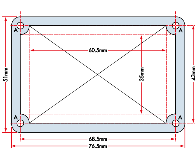
Rysunek 13 (po prawej). Dokładne wymiary wycięcia pod moduł OLED nie mają kluczowego znaczenia, ponieważ jego krawędzie nachodzą na obszar otworu na około 4 mm. Niemniej, w przypadku obudowy metalowej może być konieczne zastosowanie taśmy piankowej lub podobnego materiału w celu ochrony tylnej strony płytki drukowanej
