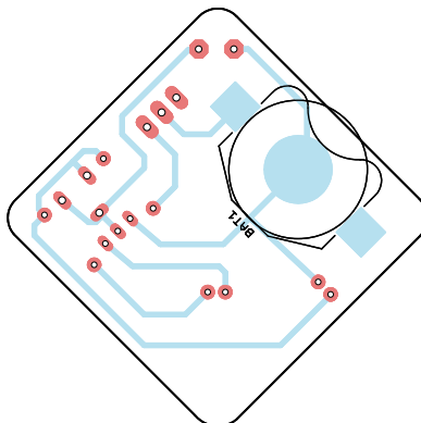
Rysunek 2. Schemat montażowy układu. Uchwyt baterii to element do montażu powierzchniowego (SMD), który należy zamontować po stronie lutowania, pozostałe elementy do montażu przewlekane (THT) należy zamontować po stronie przeciwnej
