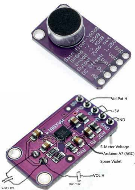
Rys. 6. Szkic podłączenia modułu AGC z układem MAX9814
