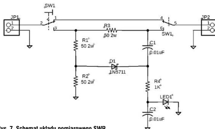
Rys. 7. Schemat układu pomiarowego SWR
