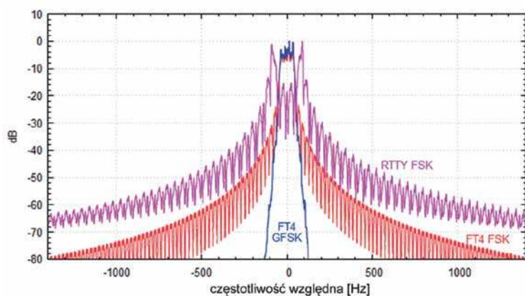
Rys. 4. Widma sygnału FT4 (niebieska krzywa) i standardowego kluczkowania FSK z zachowaniem ciągłości fazy dla tego samego komunikatu. Widmo sygnału GFSK ma szerokość 75 Hz na poziomie -6 dB, 200 Hz na poziomie -60 dB i 260 Hz na poziomie -80 dB. Dla porównania wykreślono także widmo sygnału RTTY
