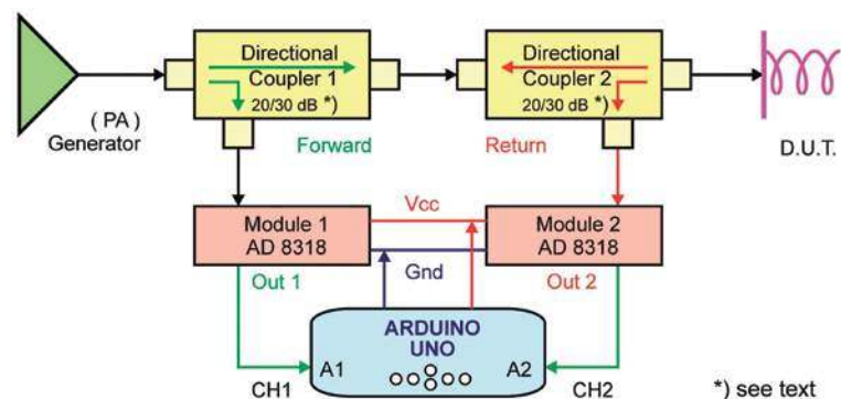
Rys. 3. Układ do pomiaru anteny
