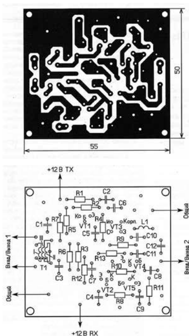
Rys. 7. PCB i rozmieszczenie elementów na płycie
