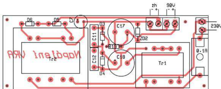
Rys. 3. Płytką drukowaną zasilacza
