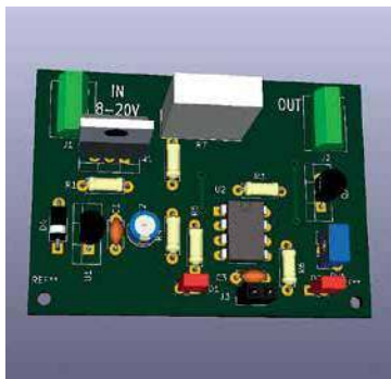
Rys. 3. Rozmieszczenie elementów na płycie drukowanej
