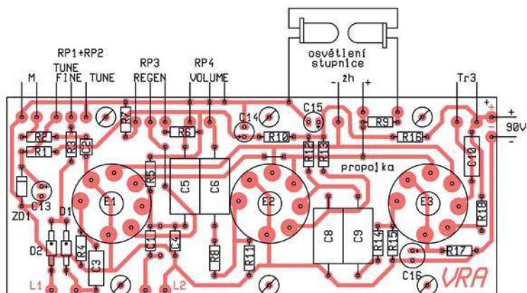
Rys. 2. Płytką drukowaną odbiornika
