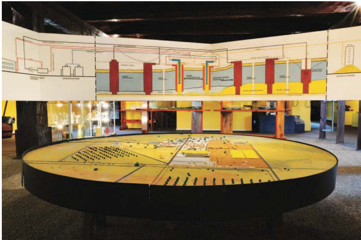
Schemat podziemnego wytopu siarki metodą Frascha, którą na wielką skalę zastosowano w Kopalni Otworowej w Jeziórku w latach 1967 – 2001
