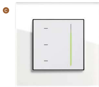
🔌 W sprzedaży znajdziemy ściemniacze przyciskowo-obrotowe (a, b) oraz dotykowe (c). Zaawansowane urządzenia zapamiętują ostatnie ustawienia natężenia światła. OSPEL, GOVENA, GIRA
