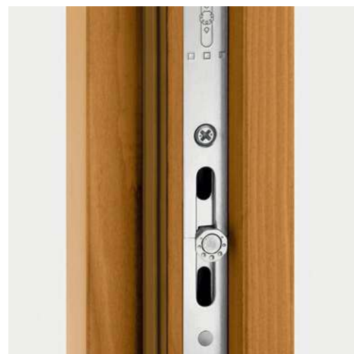
Rolka ryglująca to element okucia, będącego podstawowym antywłamaniowym zabezpieczeniem okna. WINKHAUS
