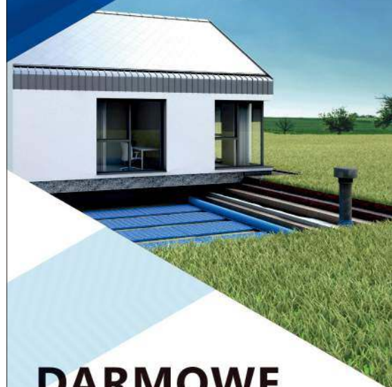
Układanie hydroizolacji na ociepleniu płyty fundamentowej.
