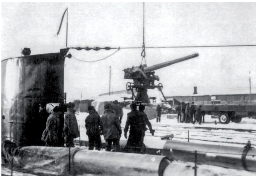
▲ Okręty podwodne Vetehinen , Vesihisi i Iku-Turso uzbrojone były także w półautomatyczną armatę kalibru 76,2 mm ULK firmy Bofors (w Finlandii oznaczoną jako 76/48 28 LT), zamontowaną na okrętach w latach 1930–1931. Można było z niej prowadzić ogień do celów morskich i powietrznych. W trakcie wojny zimowej działa zostały zdemontowane.
