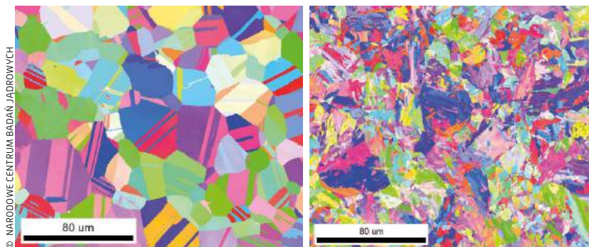
Po lewej, zoptymalizowana mikrostruktura stopu z dobrze uwidocznionymi ziarnami, poddana wyżarzaniu w wysokiej temperaturze. Po prawej, mikrostruktura badanego stopu po wytopie przed zastosowaniem obróbki termicznej.
