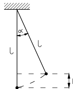
Rys. 6. Schemat do obliczania wysokości h wznesienia kulki po zderzeniu, zwieszonyj na nici o długości l , odchylonyj o kąt \alpha .
