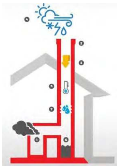
Rysunek 3. Regulator Ciągu Kominowego – system grzewczy bez regulatora: 1 – duże zużycie opału, 2 – duży poziom emisji zanieczyszczeń do atmosfery, 3 – zawiewanie, czyli cofanie spalin, 4 – praca systemu zależna od warunków pogodowych, 5 – zimny komin uniemożliwiający prawidłową pracę systemu, 6 – znaczna ilość kondensatu, 7 – erozja komina spowodowana zawilgoceniem komina
