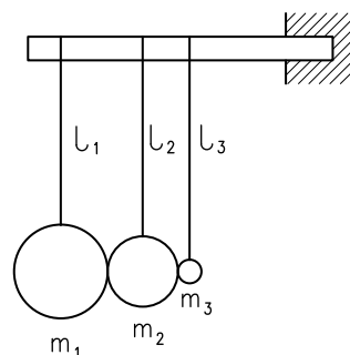
Rys. 12. Układ trzech kulek o masach m_1 , m_2 , m_3 , zawieszonych na niciach o długościach l_1 , l_2 , l_3 , przeznaczony do uzyskania wielokrotnego wzrostu prędkości po odbiciu ostatniej kulki o masie m_3 . Masy kulek powinny spełniać warunek m_1 \gg m_2 \gg m_3 .
