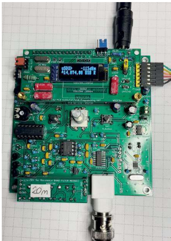
TRX \mu SDX w wyświetlaczu OLED
