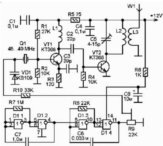
Rys. 4. Schemat radiolatarni (bikony) FM/2 m
