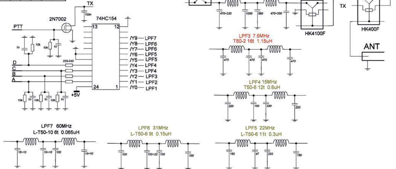
Rys. 3. Schemat ideowy modułu filtrów LPF
