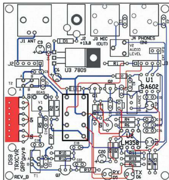
Rys. 2. Rozmieszczenie elementów na płycie TRX-a
