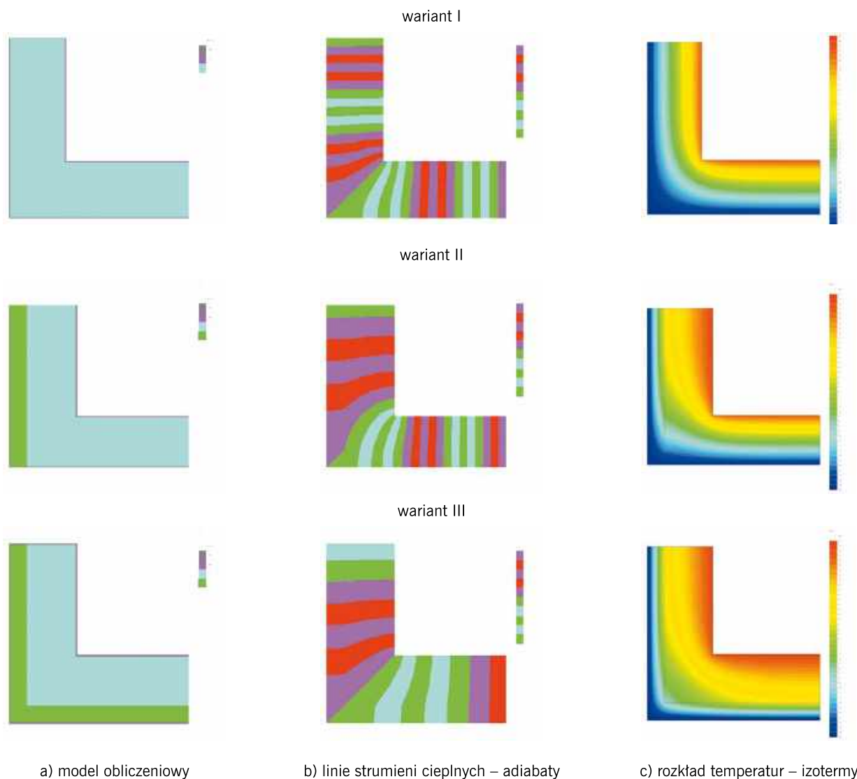
RYS. 1 Połączenie ścian zewnętrznych w narożniku przed i po dociepleniu: a) model obliczeniowy, b) linie strumieni ciepłych – adiabaty, c) rozkład temperatury – izotermy – opracowanie własne
