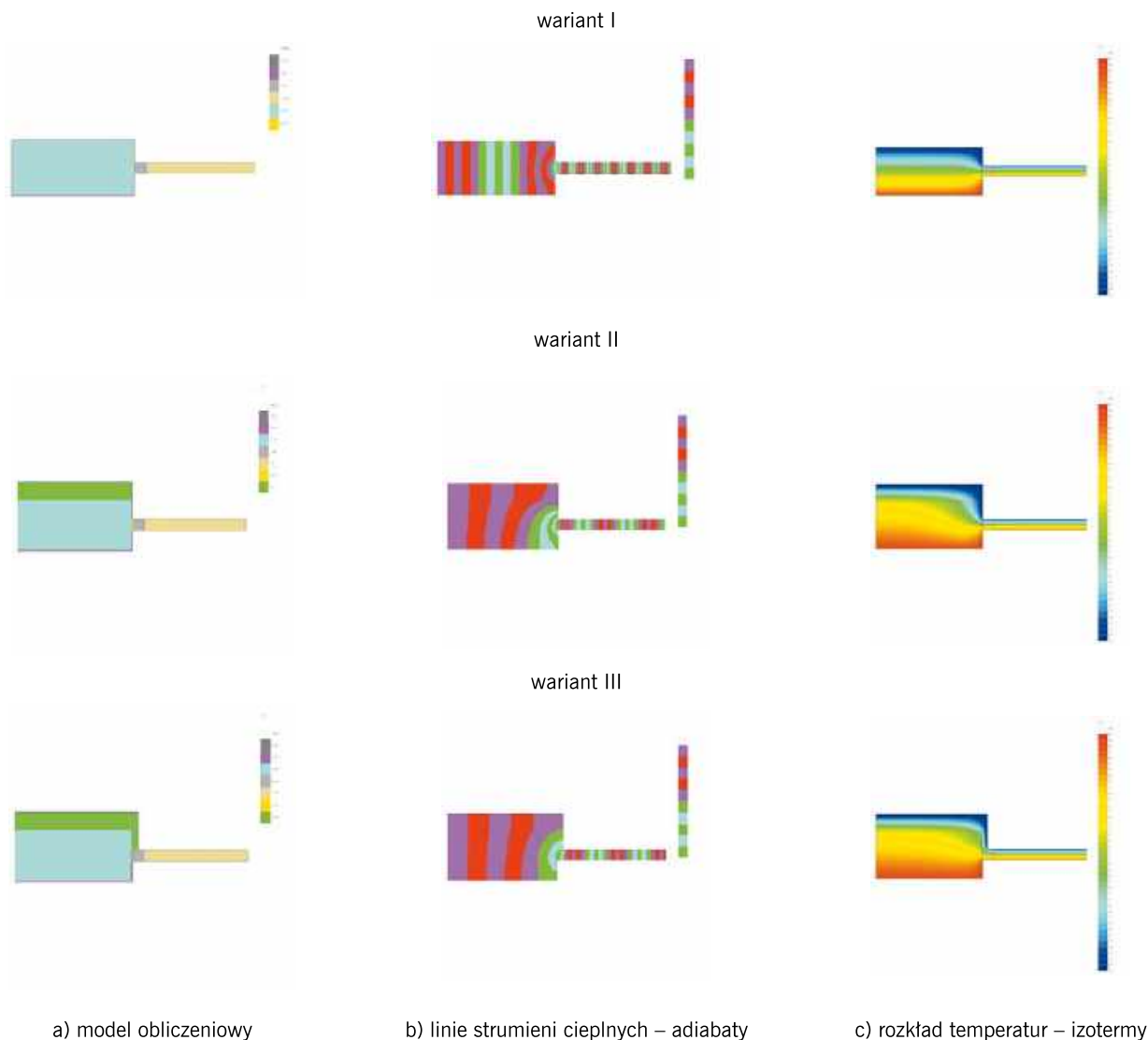
RYS. 2 Połączenie ściany zewnętrznej z oknem w przekroju przez ościeżnicę przed i po dociepleniu: a) model obliczeniowy, b) linie strumieni ciepłych – adiabaty, c) rozkład temperatury – izotermy – opracowanie własne
