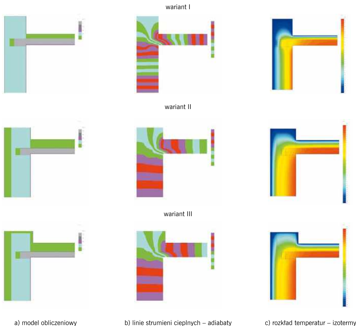
RYS. 3 Połączenie ściany zewnętrznej ze stropodachem przed i po dociepleniu: a) model obliczeniowy, b) linie strumieni ciepłych – adiabaty, c) rozkład temperatury – izotermy – opracowanie własne
