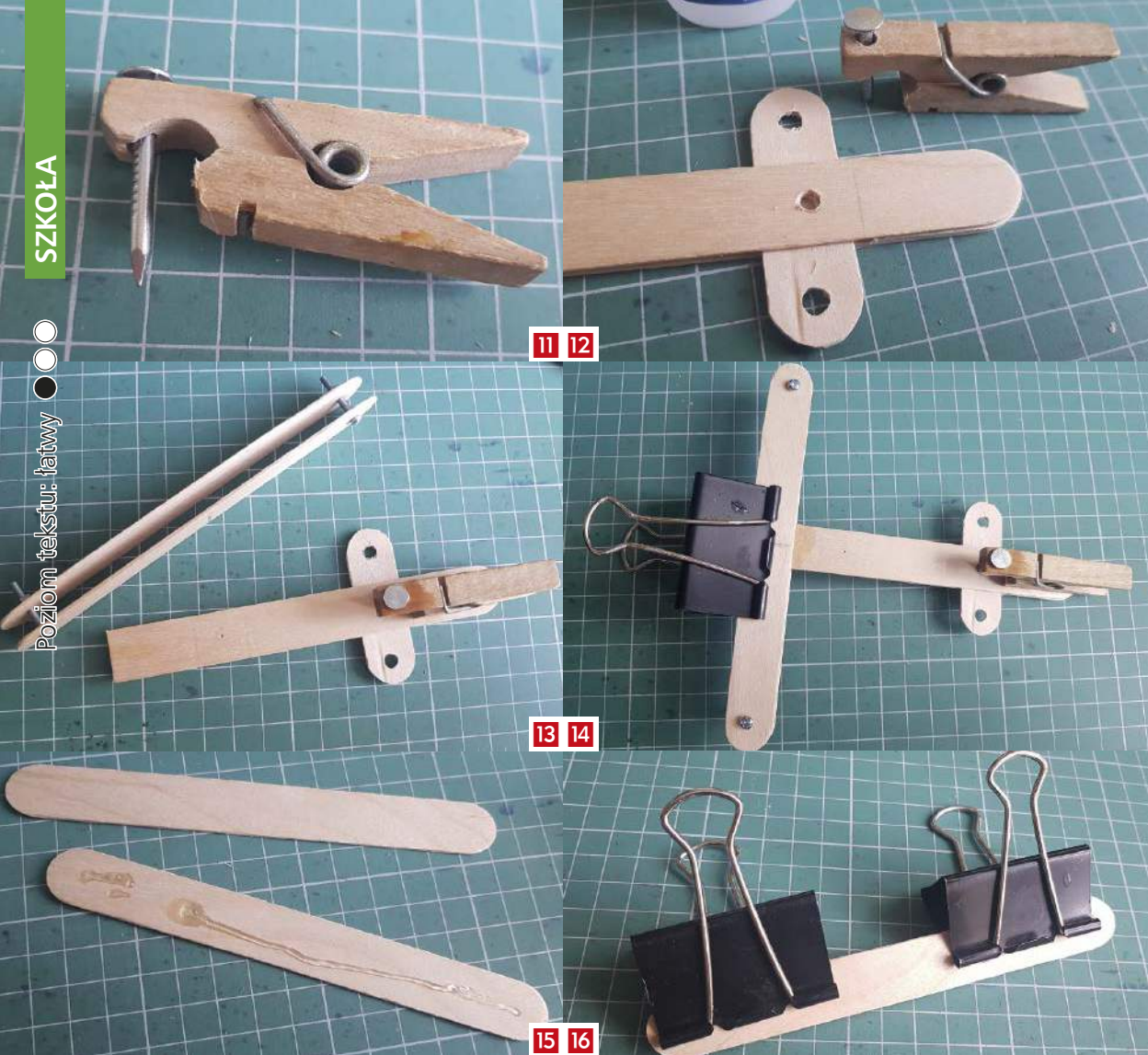
11. Spust kuszy z gwoździem; 12. Zamek i spust kuszy przed sklejeniem; 13. Gwóźdź ma trafić w otwór i zaczepiać o zamek; 14. Doklejanie ramion; 15. Niewielka ilość cyjanowego kleju wystarczy; 16. Klejenie uchwytu
