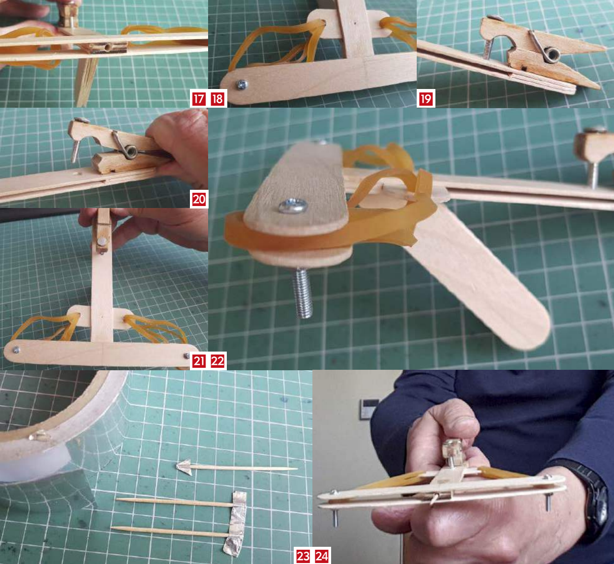
17. Rozwierzony wylot kuszy; 18. Zamontowane cięciwy; 19. Gwóźdź opiera się o dolną ściankę korpusu; 20. Sprawdzamy działanie; 21. Teraz wystarczy napiąć cięciwę; 22. Widok kuszy z boku; 23. Przygotowanie bełtów; 24. Kusza gotowa do strzału
