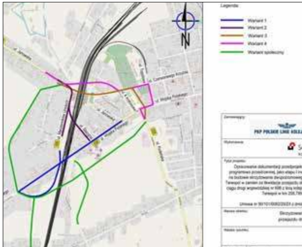
Plan orientacyjny 5 wariantów budowy tunelu, z uwzględnieniem wariantu społecznego (nr 5) budowy wiaduktu w Terespolu
