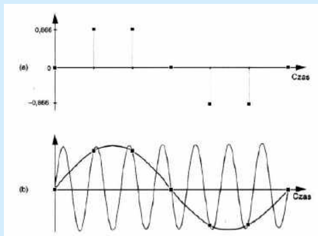
Rysunek 36. Ilustracja zjawiska niejednoznaczności częstotliwości w dziedzinie czasu [2]
