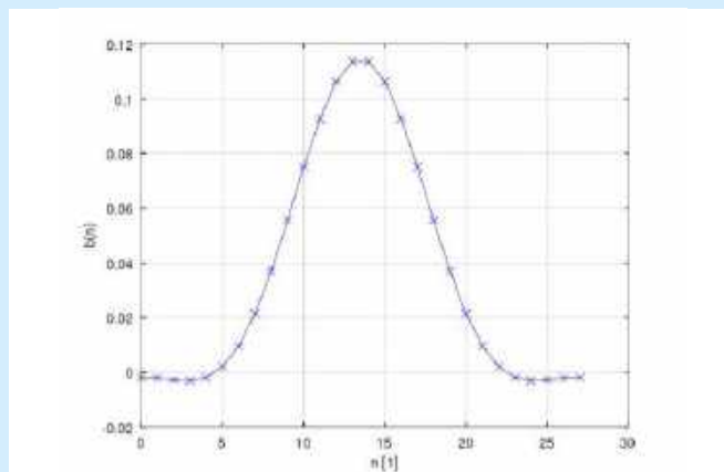
Rysunek 43. Współczynniki b(n) filtru FIR LPF
