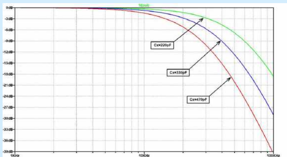
Rysunek 40. Charakterystyki częstotliwościowe prototypu filtrów analogowych
