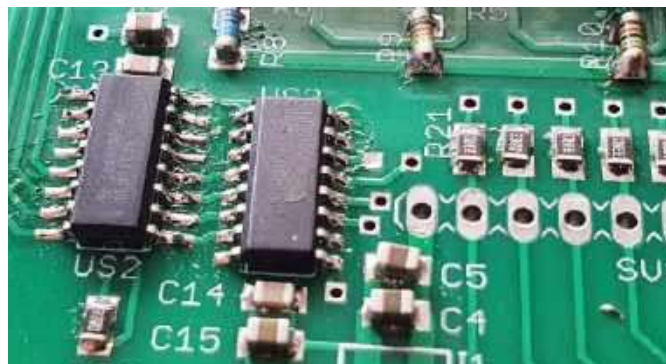
Fotografia 3. Inny układ 74HC595, który również został uszkodzony zbyt wysokim napięciem zasilającym
