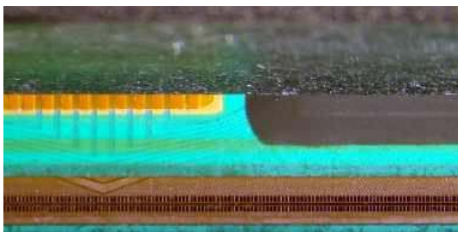
Fotografia 4. Makrofotografia przykładowej głowicy termicznej. Czarny, zaokrąglony element w prawej części zdjęcia to warstwa epoksydu, którym zalano układ COB współpracujący z głowicą
