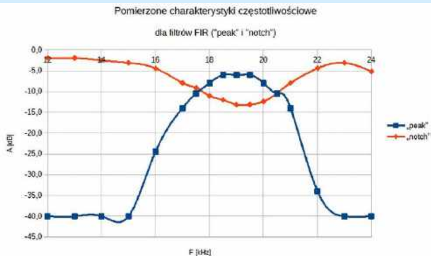
Rysunek 54. Zmierzone charakterystyki częstotliwościowe filtrów FIR (peak i notch)
