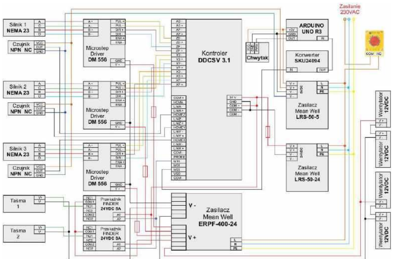
Rysunek 4. Schemat ideowy układu sterowania robota kartezjańskiego
