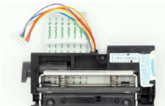
Fotografia 11. Popularny model mechanizmu termicznego, stosowany m.in. w przenośnych kasach fiskalnych. Doskonale widoczne są: czujnik obecności papieru oraz docisk sprężynowy w metalowej ramie, pełniący jednocześnie rolę mocowania wałka napędowego. W tym modelu silnik, czujnik papieru oraz czujnik wałka są podłączone za pomocą wiązki pojedynczych przewodów, zakończonej złączem rastrowym, zaś taśma FFC obsługuje jedynie głowicę termiczną
