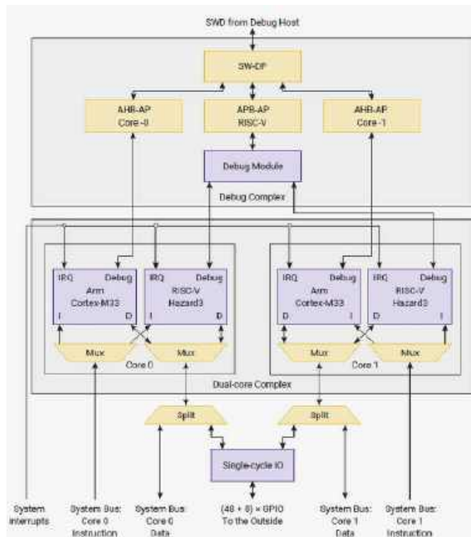
Rysunek 2. Architektura podsystemu procesora układu RP235x [6]
