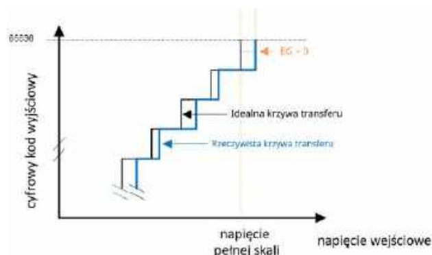
Rysunek 27. Błąd wzmacnienia
