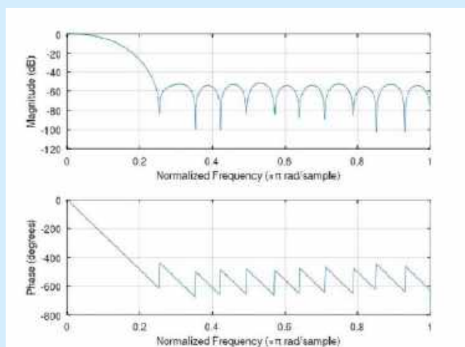
Rysunek 44. Charakterystyki: amplitudowa i fazowa filtru FIR LPF (symulacja)
