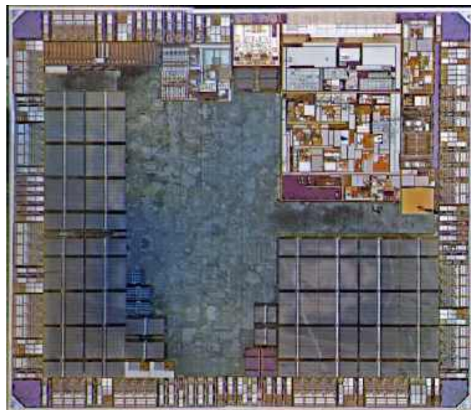
Fotografia 1. Warstwa dyfuzyjna procesora RP2350 [2]
