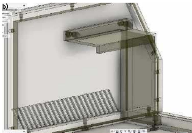
Rysunek 7. Osłona radiatora: sam element (a) i osłona z panelami, do których będzie umocowana (b)
