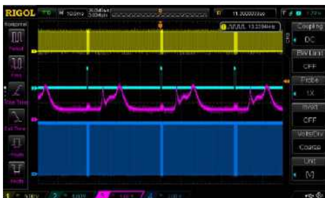
Rysunek 7. Oscylogram zarejestrowany podczas wykonywania kilku kolejnych akwizycji za pomocą minispektrometru marki Hamamatsu. Poziomy szum w sygnale wideo wynika z zastosowanego układu aplikacyjnego, użytego tylko do szybkiej oceny działania spektrometru (płytkę z mikrokontrolerem była zasilana bezpośrednio z portu USB, co wpłynęło na poziom szumów impulsowych w całym układzie)
