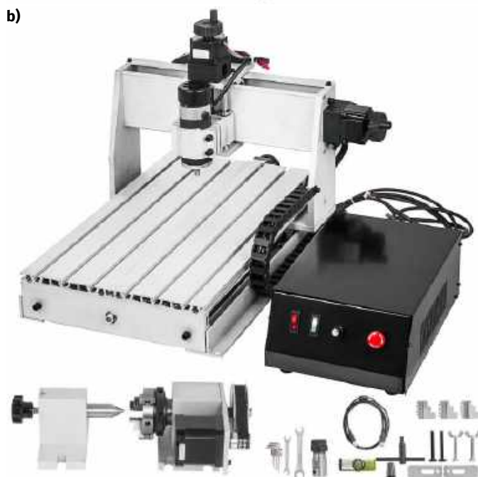
Fotografia 30. Frezarki CNC 3020 (a) i 3040 (b). Oferują najlepszy stosunek ceny do możliwości
