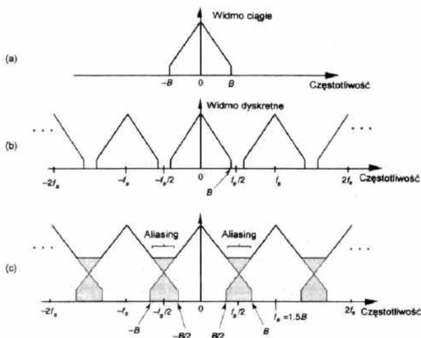
Rysunek 35. Ilustracja zjawisk powielania widmowego i aliasingu [2]
