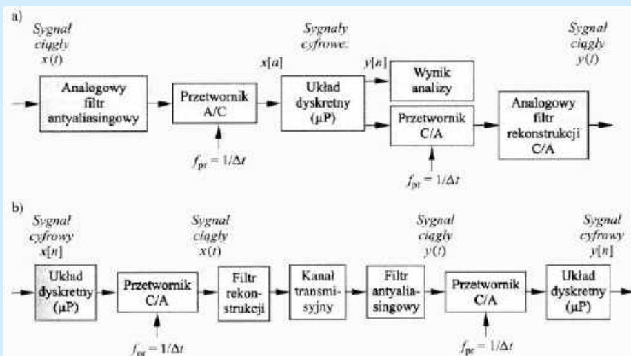
Rysunek 34. Cyfrowe torów analizy i przetwarzania sygnałów analog-cyfra-analog oraz cyfra-analog-cyfra [1]
