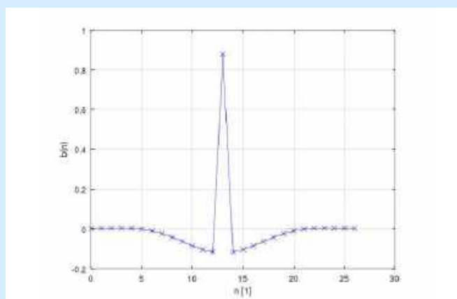
Rysunek 45. Współczynniki b(n) filtru FIR HPF
