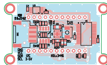
Rysunek 3. Rozmieszczenie elementów na PCB
