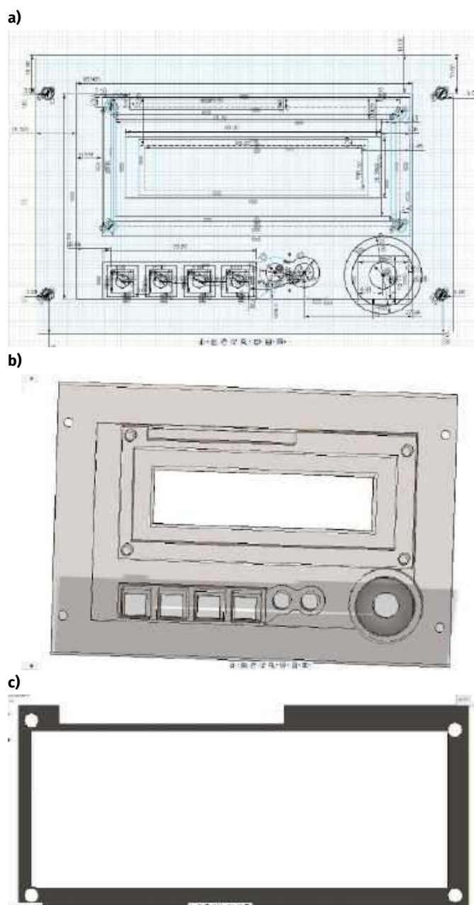
Rysunek 10. Panel kontrolny: szkic (a), gotowy model (b) i element dystansowy między wyświetlaczem a płytką drukowaną panelu (c). Jest to najbardziej skomplikowany komponent obudowy – na szkicu odtworzono wszystkie wymiary płytki drukowanej i wyświetlacza
