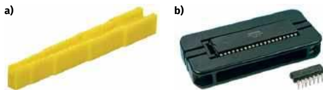
Fotografia 19. Przystawki do doginania wyprowadzeń komponentów osiowych (a) i układów scalonych (b)
