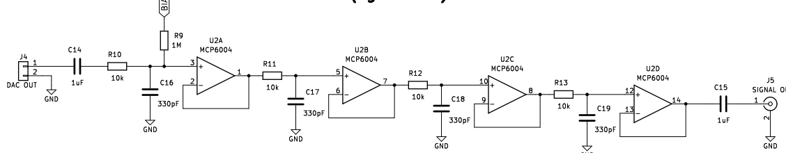
Rysunek 42. Schemat elektryczny analogowych układów filtrujących
