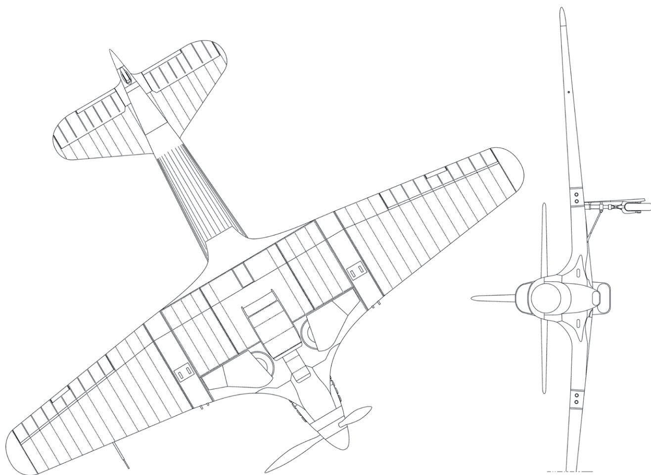
Renard R.40, rysunek przedstawiający finalny etap rozwoju belgijskiej rodziny myśliwców. Widoczne rzuty (boczny, górny, dolny i czołowy) dokumentują unikalną sylwetkę samolotu z gładką linią grzbietową kadłuba i zoptymalizowanym układem chłodzenia.
