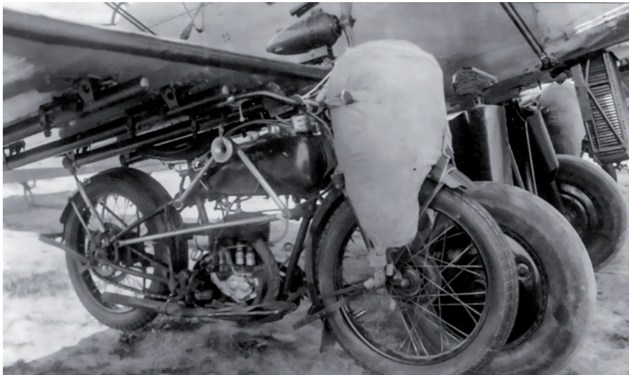
▲ Widok z boku na samolot R-5 z 3. Brygady Lotniczej Specjalnego Przeznaczenia z dwoma podwieszonymi motocyklami. W odróżnieniu od systemów G-9 i G-36 spadochron jest umieszczony nie w metalowym a w miękkim pojemniku umieszczonym przed pojazdem.
