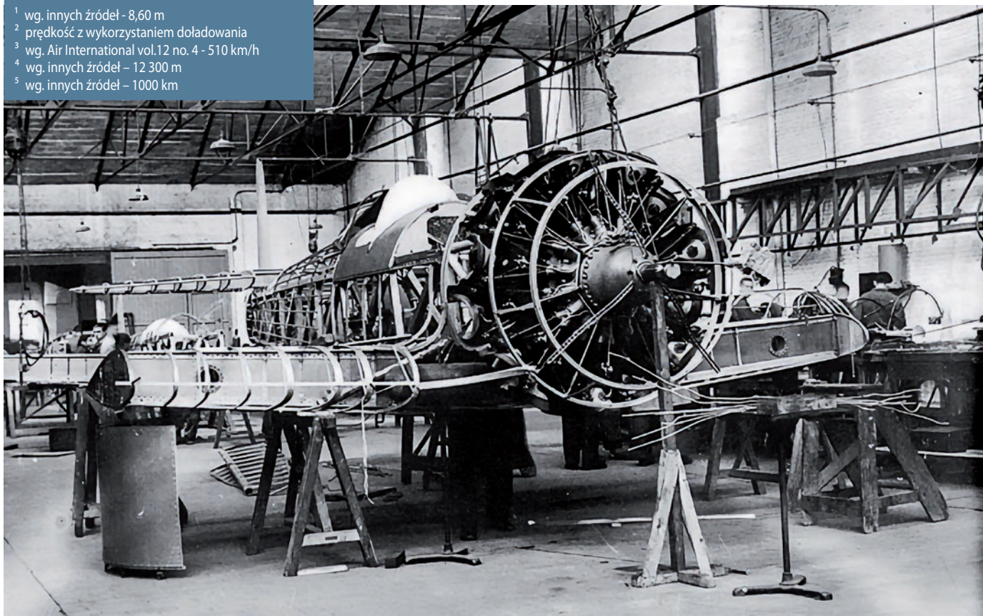
▼ Prototyp Renard R.37 w trakcie budowy.
