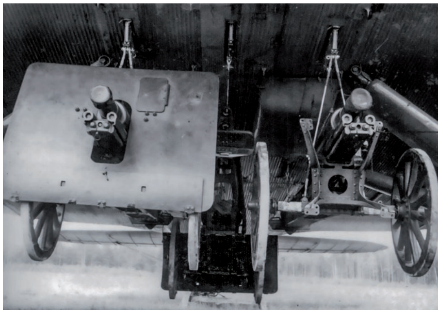
▲ Trzy 76 mm armaty górskie wzór 1913 rok umieszczone pod samolotem TB-3 na systemie podwieszenia opracowanym przez CBOI CAGI. Dwa działa są zawieszane lufami w kierunku lotu a jedno w położeniu odwrotnym. Egzemplarz po prawej stronie ma zdjętą tarczę ochronną, bowiem te elementy w trakcie lotu uderzały o siebie i konstrukcję płatowca. Zdjęcie wykonano podczas prób systemu w czerwcu 1936 roku.
