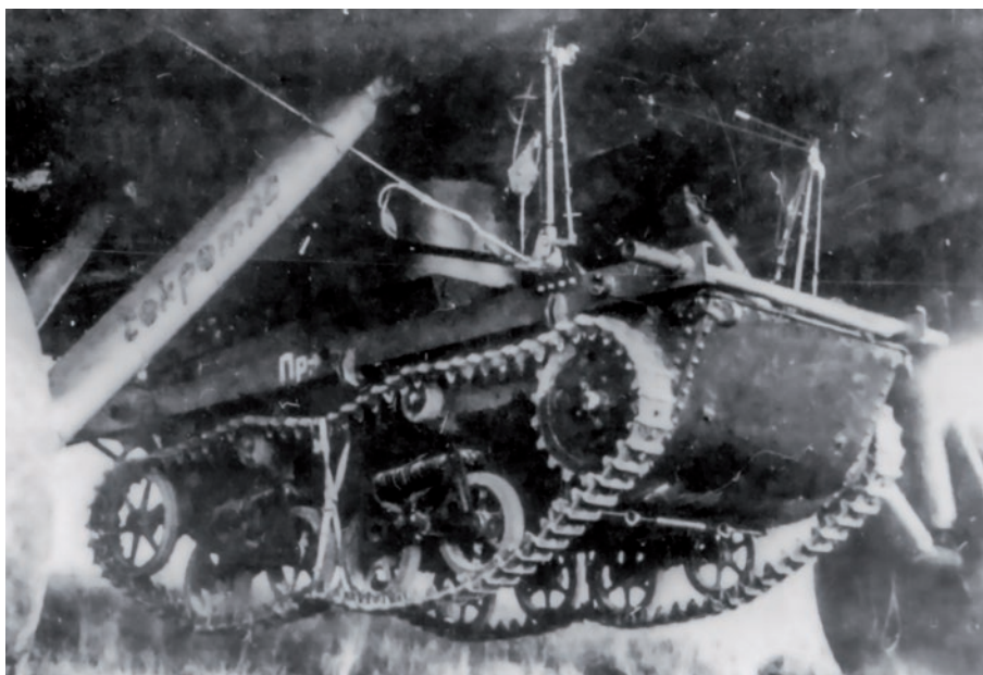
▲ Lekki czołg pływający T-37A podwieszony na systemie PG-12 pod samolotem TB-3. Do testów czołg ma zdemonstrowane boczne drewniane płytki a gaśienice są zabezpieczone przed spadnięciem.
