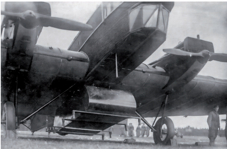
▲ Pojemnik transportowy PD-M2 o ładowności 1000 kg podwieszony pod samolotem bombowym TB-1. Wewnątrz były przewożone dwa motocykle z koszami. Pod pojemnikiem widać wykonane z rurek podstawki.
