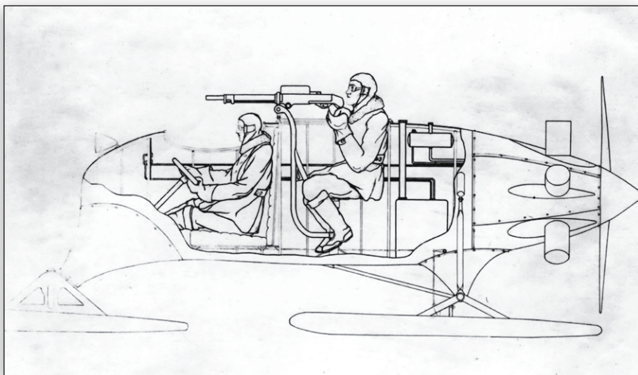
▲ Wykonany chyba przez samego Grochowskiego rysunek przedstawiający proponowany pojazd bojowy na płozach. Widać rozmieszczenie członków załogi i uzbrojenia. Za strzelcem widać zbiorniki paliwa i oleju. Aerosanie miały być zrzucone razem z załogą bezpośrednio na grubą warstwę śniegu. Trudno powiedzieć, czy było to realne.
