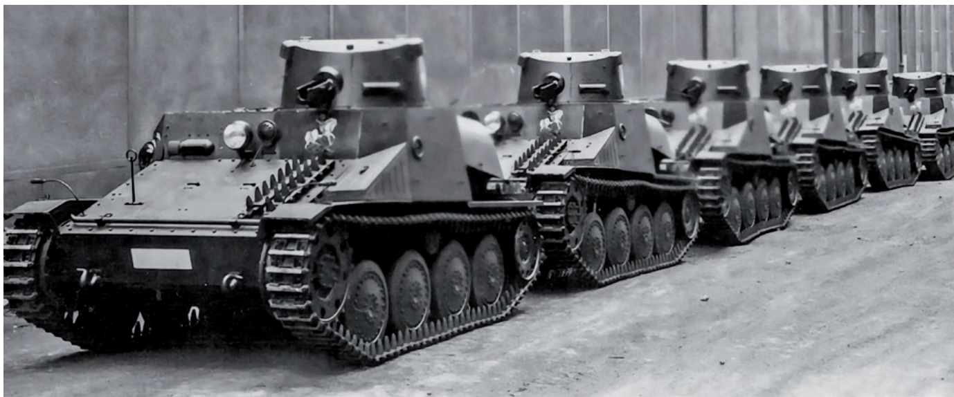
▲ Gotowe do wysłania czołgi Praga AH-IVHB w marcu 1950 r. Ważnym argumentem przy okazji podjęcia decyzji o nabyciu tego sprzętu przez Etiopię okazały się prezenty, w tym np. kryształowe lustra, luksusowa broń myśliwska, które trafiły w m.in. w ręce samego cesarza Hajle Syllasje.
