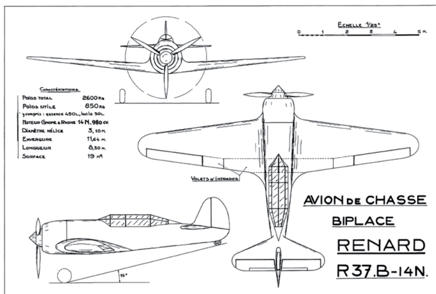
◀ Szkic samolotu Renard R.37B.
