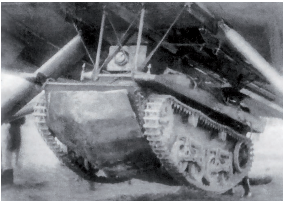
▲ Czołg pływający T-37A na podwieszeniu TWD-2 pod samolotem TB-3. Jak widać do testów zdemontowano karabin maszynowy. W tym czołgu chyba skrócono taśmy gąsienic bowiem nie widać silnego zawisania.
