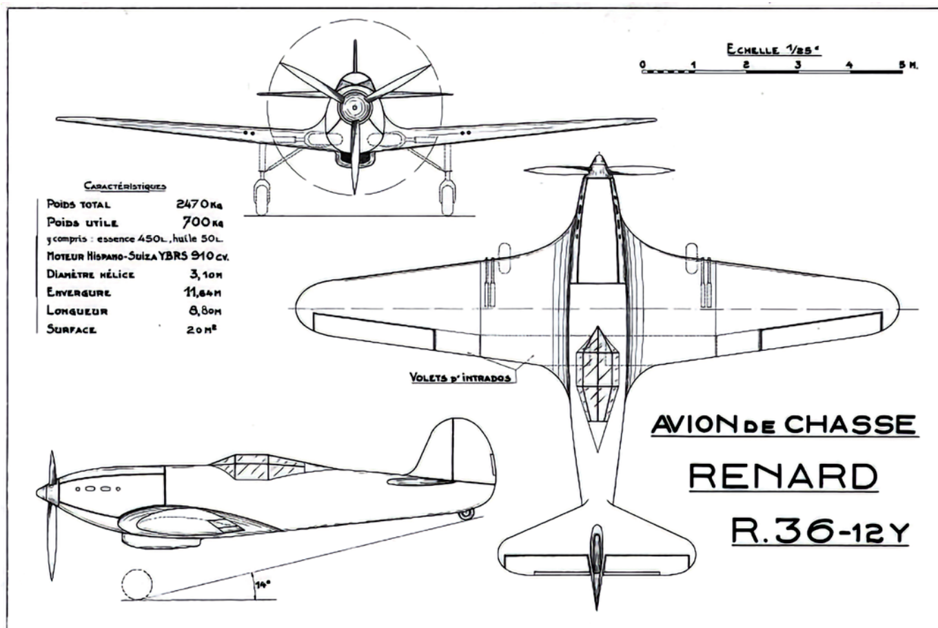
▼ Rysunek wstępny samolotu R-36.
