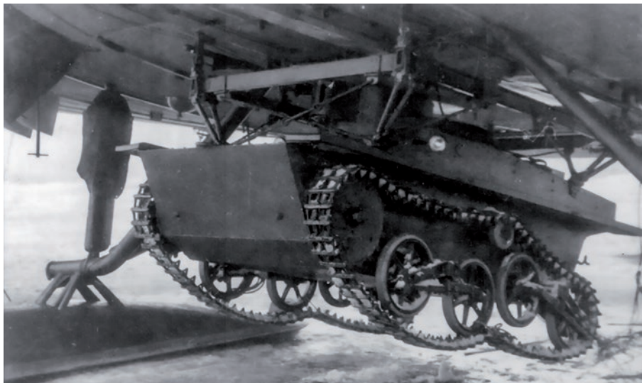
▲ Seryjny czołg T-41 podwieszony pod samolotem TB-3. Jak widać testy były prowadzone w okresie zimowym, bowiem podwozie płatowca jest wyposażone w płozy. Zwisające gaśienice są przymocowane do kół jezdnych, co może wskazywać, że testowano jedynie system podwieszania z dość masywną ramą umieszczoną pod kadłubem TB-3. Przy pokrywie lodowej na zbiornikach wodnych zrzucanie czołgu raczej mogło być niemożliwe.
