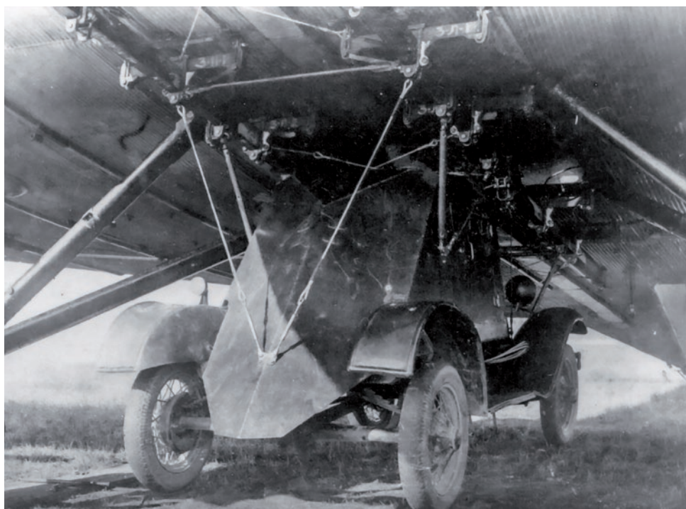
▲ Samochód pancerny D-12 na podwieszeniu PG-12 pod samolotem TB-3. Wymiary pojazdu wymuszały podwieszenie tyłem do kierunku lotu. Tu dobrze widać, że na pancerzu tylnej części przedziału bojowego został umieszczony zaczep cięgien stabilizujących samochód w trakcie lotu.
