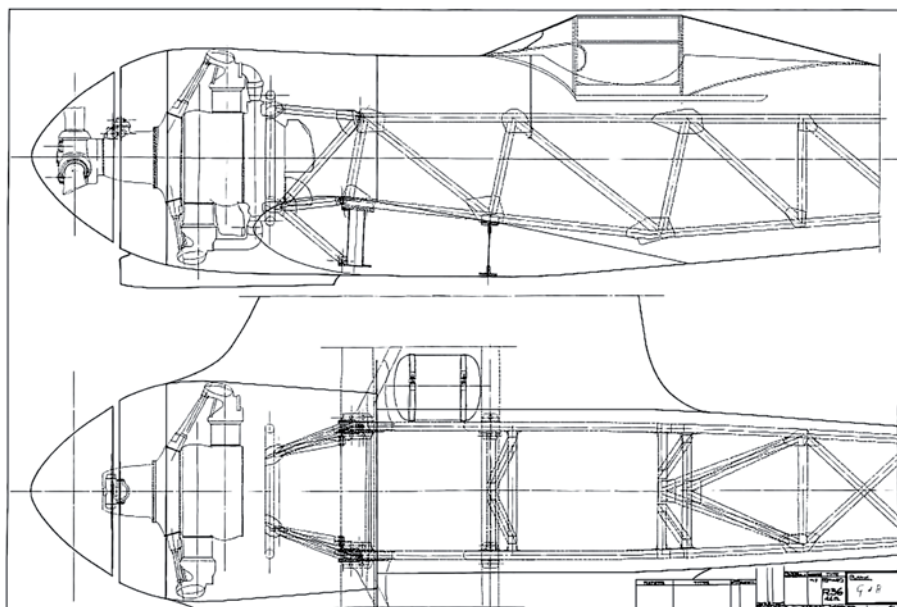
▲ Rysunek instalacji silnika w kadłubie samolotu Renard R.37.
