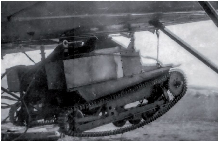
▲ Tankietka T-27 podwieszona pod samolotem TB-3 z wykorzystaniem systemu opracowanego przez OTKB. System ten wykluczający zrzut na spadochronie mógł służyć jedynie do transportu.
