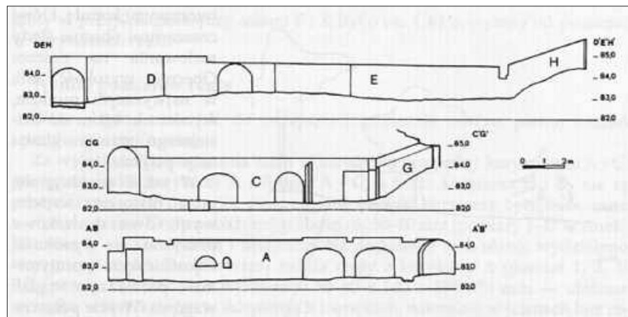
Ryc. 2. Wzgórze Abrahama. Przekrój podłużny korytarzy A, C, D-E-H (oprac. D. Stabrowska)
