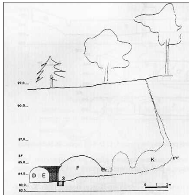
Ryc. 2a. Przekrój poprzeczny przez: korytarz D-E, salę F oraz rekonstrukcję sali K i szybu (oprac. D. Stabrowska)
