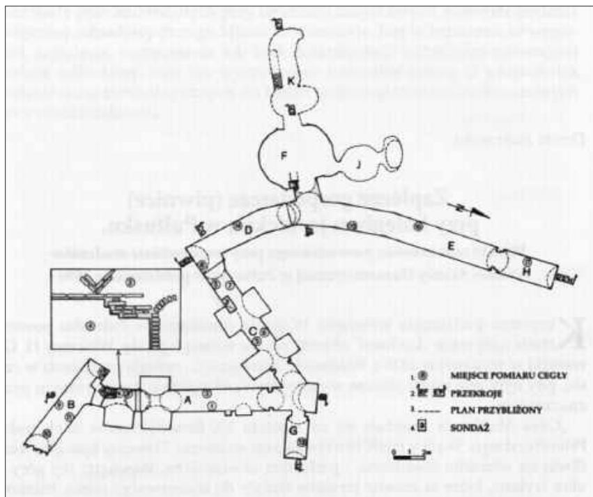
Ryc. 1. Wzgórze Abrahama. Plan podziemnych korytarzy. Oznaczenie miejsc: pomiaru cegły, przekrojów, sondazy archeologicznych (1-3), przybliżonego zasięgu niebadanych części korytarzy (oprac. D. Stabrowska)
