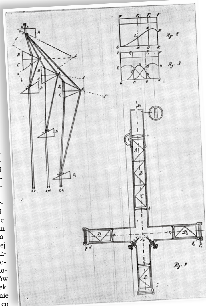
Schemat rozszczepiania światła i opis patentowy projektu budowy kamery
