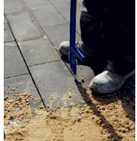
3 Wypełnienie piaskiem szczelin między kostkami to kluczowy etap prac, który stabilizuje całą nawierzchnię i chroni bruk przed przesuwaniem się podczas użytkowania. POLBRUK
