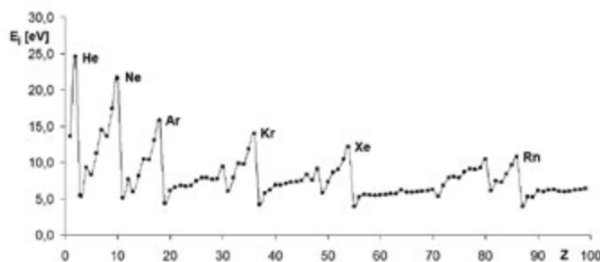
Rys. 2. Wykres pierwszej energii jonizacji pierwiastków w funkcji ich liczby atomowych to również przykład okresowych zmian własności pierwiastków.
