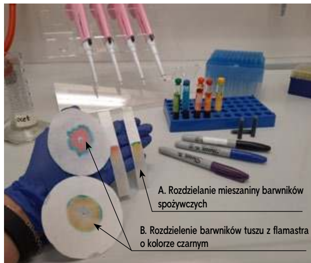
Rysunek 12. Wyniki doświadczeń – barwne chromatogramy uzyskane przy rozwijaniu A – wstępującym, B – odśrodkowym.
