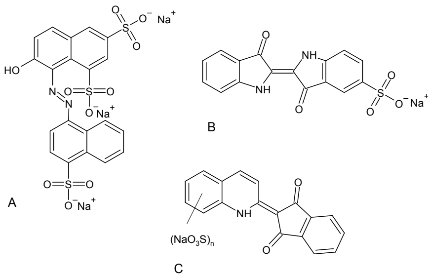
Rysunek 7. Poglądowe struktury chemiczne wybranych barwników spożywczych: A – czerwień koszenilowa (E124) – barwnik czerwony, B – indygotyna (E132) – barwnik niebieski, C – żółcień chinolinowa (E102) – barwnik żółty.
