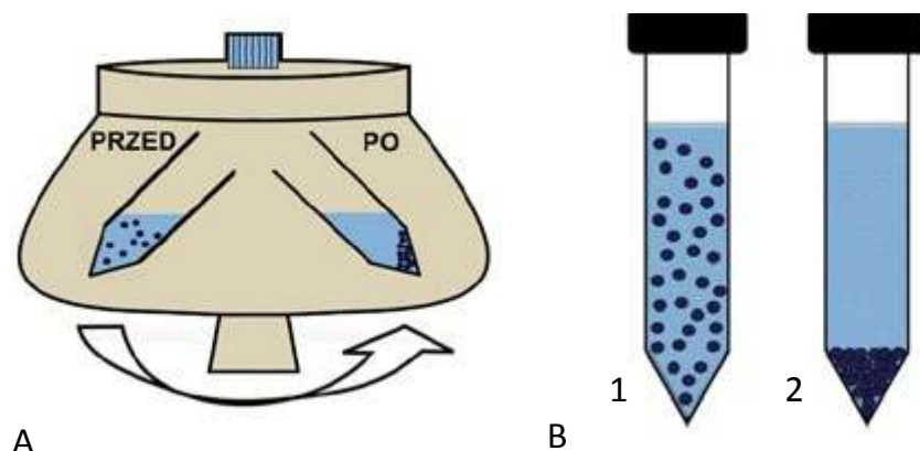
Rysunek 2. A- Schematyczna budowa wirówki laboratoryjnej; próbka umiejscowiona jest w bębnie, który jest wprawiany w ruch obrotowy w zaznaczonym kierunku B - 1. fiolka z zawiesiną przed poddaniem próbki odwirowaniu 2. ta sama fiolka po odwirowaniu próbki; osad - dolna warstwa, tzw. supernatant - górna warstwa.
