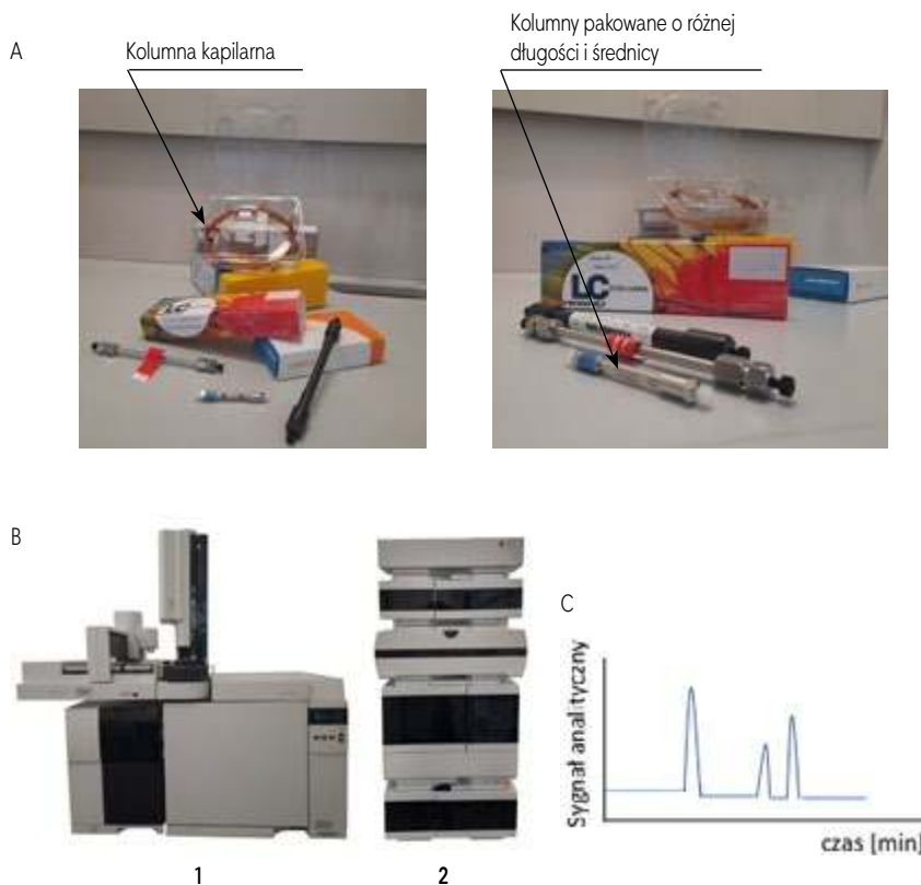
Rysunek 6. Ilustracje A – kolumna chromatograficzna (faza stacjonarna), B – chromatograf: 1 – gazowy, 2 – ciekłowy (aparatus do rozdzielania składników mieszanin jednorodnych), C – chromatogram pikowy (obraz przedstawiający efekt rozdzielania składników analizowanej próbki, na którym każdemu sygnałowi (pikowi chromatograficznemu) odpowiada konkretny składnik próbki badanej).
