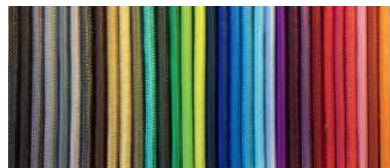
ⓘ Przewody dekoracyjne 3 x 1,5 mm 2 w oplocie z jedwabiu syntetycznego, średnica 7–8,2 mm, dostępne są w wielu kolorach. SOLVE24.PL
