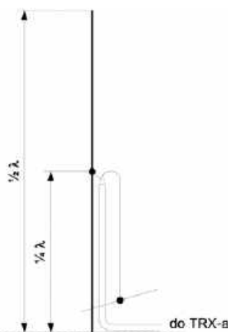
Rys. 2. Początkowa koncepcja anteny
