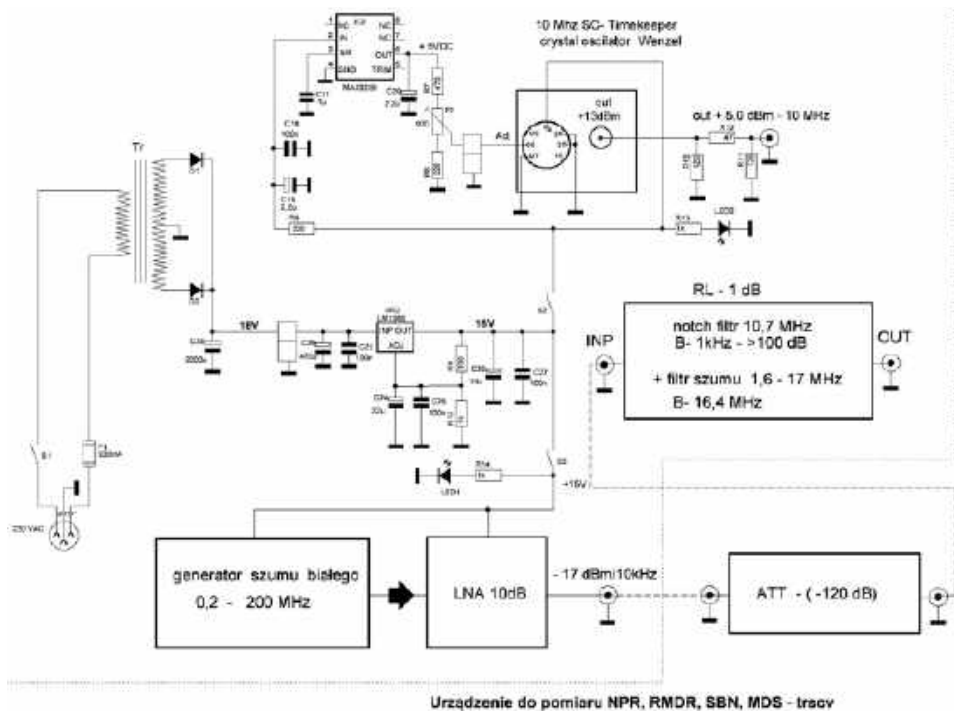
Rys. 2. Schemat blokowy przyrządu
