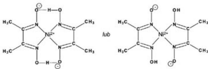
Kompleks jonów \text{Ni}^{2+} z dimetylogliksymem.
