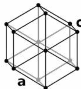
Struktura krystaliczna \alpha -Pm ( https://en.wikipedia.org/wiki/Promethium )
